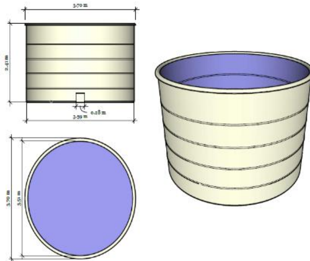
Εικόνα 2. Πλαστική υδατοδεξαμενή ανοιχτού τύπου, χωρητικότητας 25\text{m}^3 (25.000 lt) κατακόρυφου τύπου.
