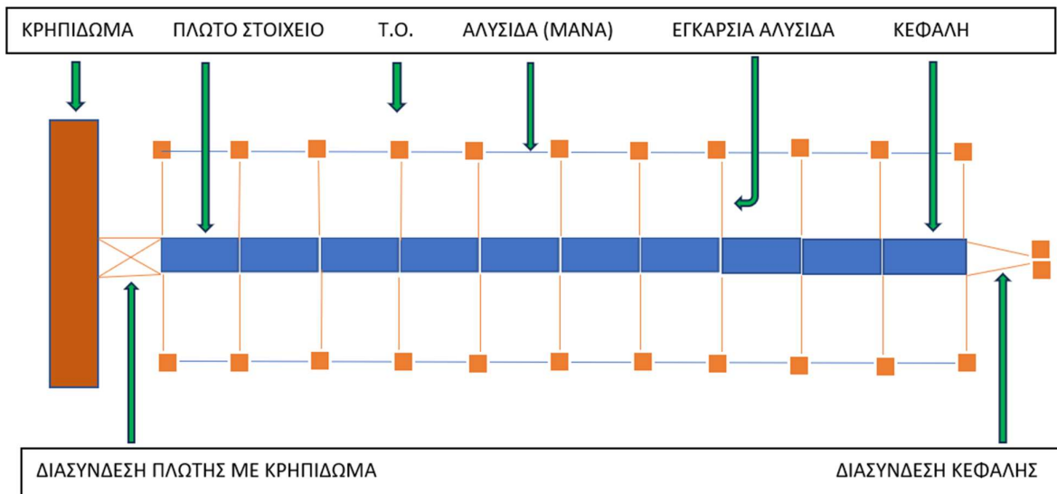
Σχ. 2 Σχεδιάγραμμα τυπικής αγκύρωσης πλωτού προβλήτα
