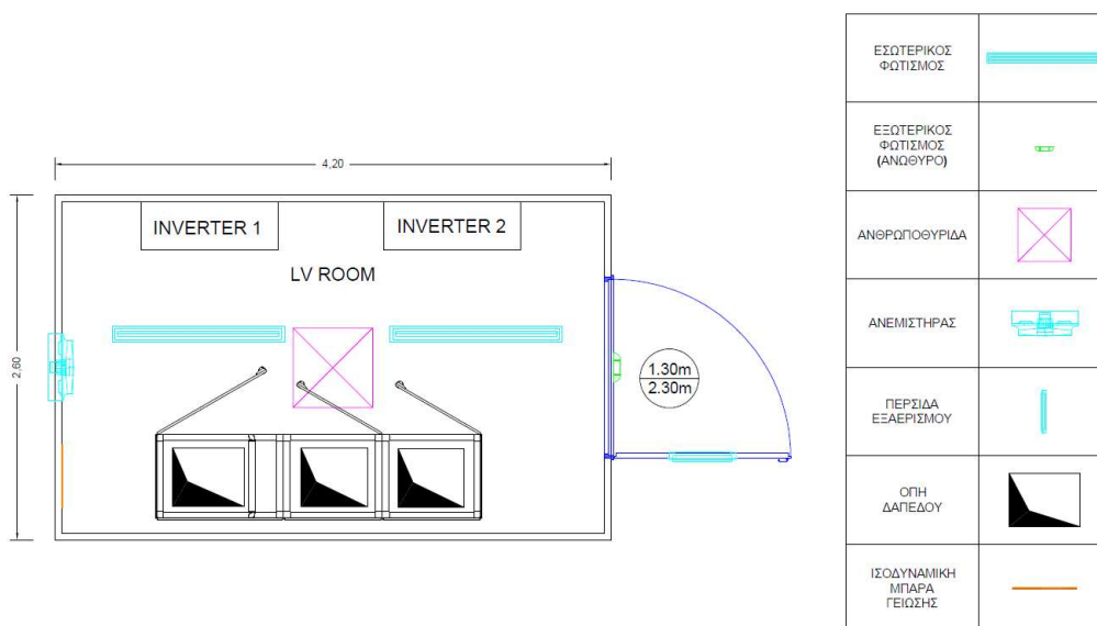
Σχ. 5 Σκαρίφημα οικίσκου
