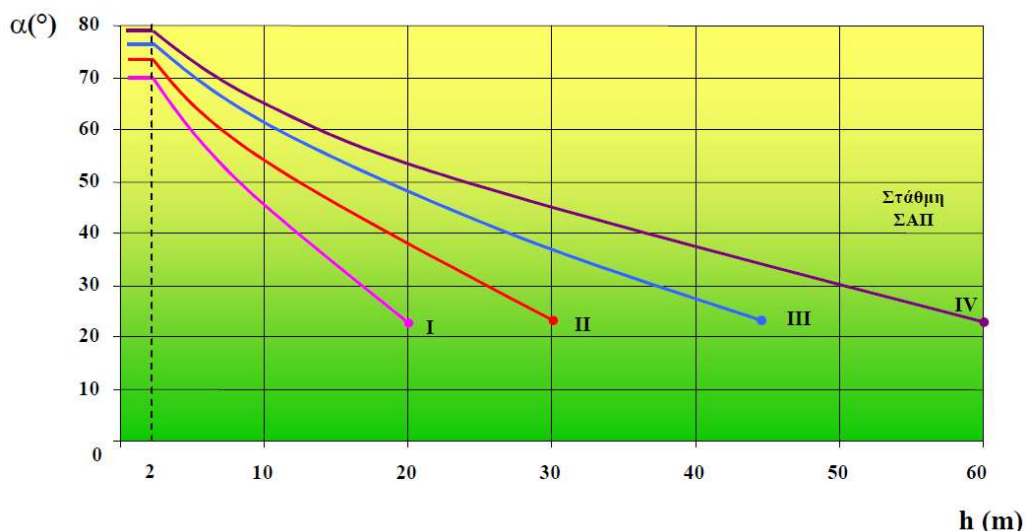
Σχ. 6 Μεση απόσταση αγωγών καθόδου
