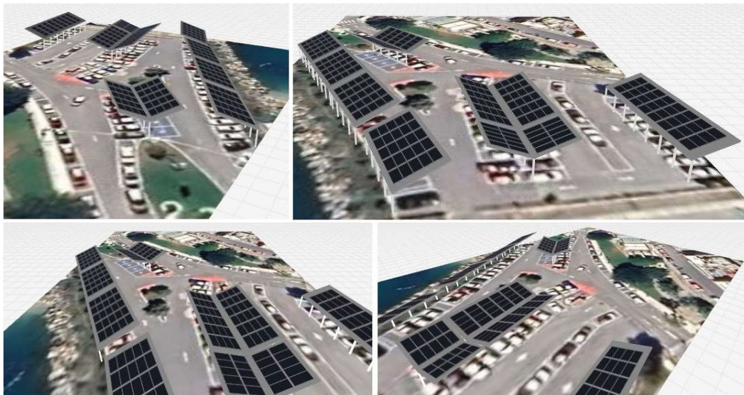
Εικόνα 4: Ενδεικτική χωροθέτηση φωτοβολταϊκού συστήματος με 240 ΦΒ πλαίσια συνολικής ισχύος 141,6 kWp.
