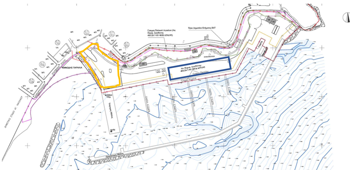
Σχ. 8 Χώρος διαχείμησης σκαφών (μπλέ περιγραμμά)
