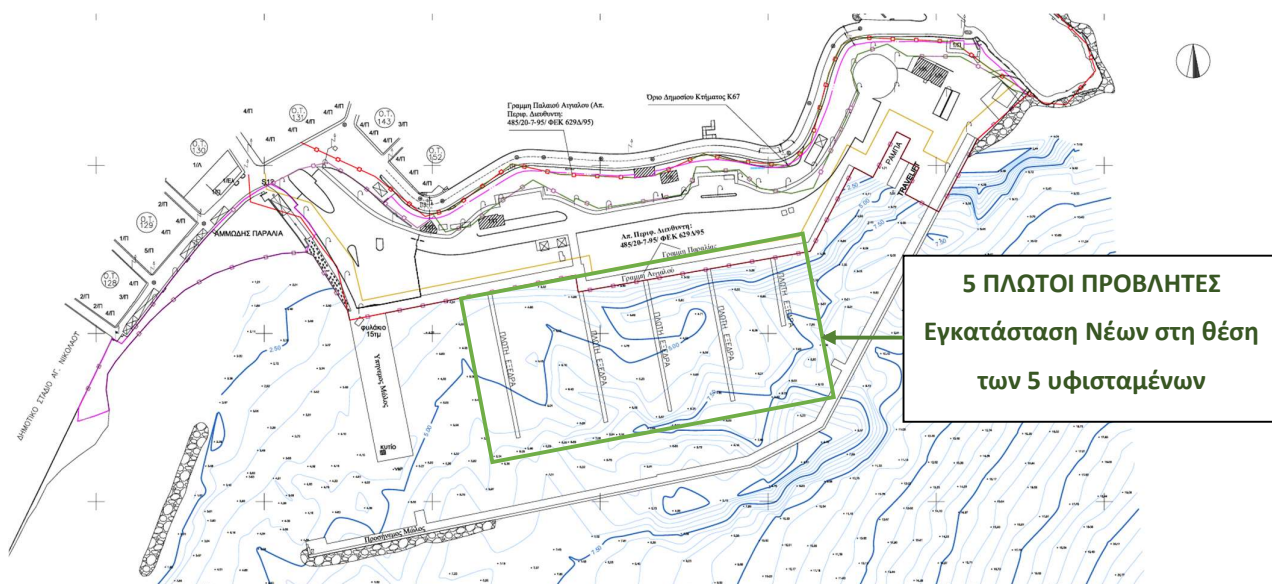
Σχ.1 Σχεδιάγραμμα της μαρίνας που φαίνονται και οι υφιστάμενοι πλωτοί προβλήτες
