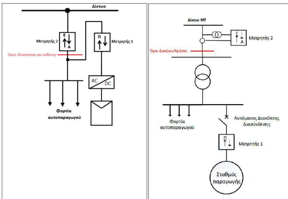
Εικόνα 3: Απλοποιημένο μονογραμμικό διάγραμμα εσωτερικής ηλεκτρικής εγκατάστασης ΧΤ και ΜΤ όπως διαμορφώνεται μετά τη σύνδεση του Πάρκου παραγωγής. Στο διάγραμμα δεν απεικονίζονται τα
