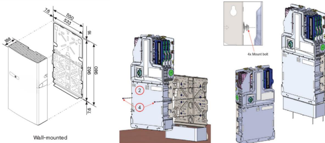
Εικόνα Γ.1-TB Μέθοδος εγκατάστασης μπαταριών.
