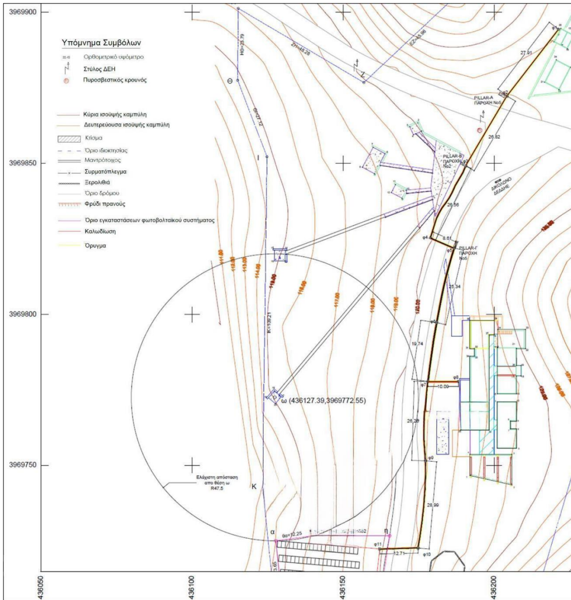
Εικόνα Γ.7-ΤΑ Η όδευση των παροχικών καλωδίων μεταξύ του γενικού πίνακα χαμηλής τάσης του ΦΒΣ και των εγκαταστάσεων του ΠΑΓΓΑΙΑ.
