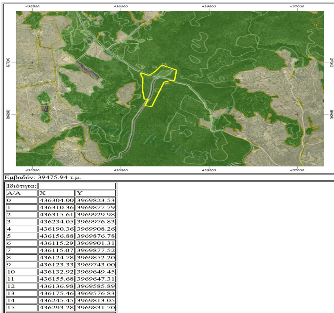
Εικόνα Γ.1-ΤΑ. Το αγροτεμάχιο που θα κατασκευαστούν οι ΦΒΣ.
