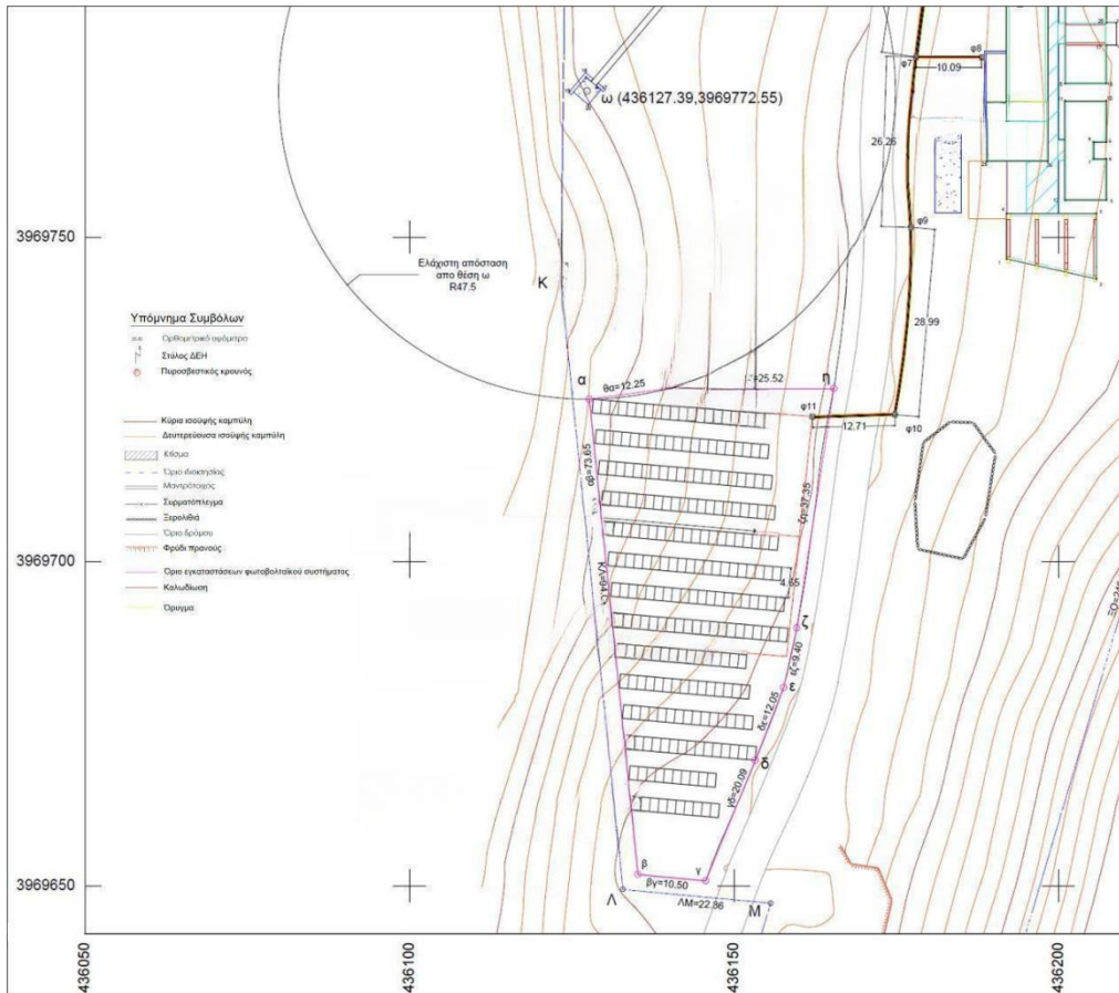
Εικόνα Γ.2-ΤΑ Ενδεικτική χωροθέτηση του ΦΒΣ.
