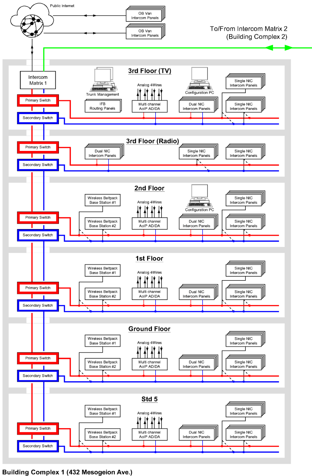
Σχήμα 1: Σχηματικό διάγραμμα συστήματος στο Ραδιομέγαρο
