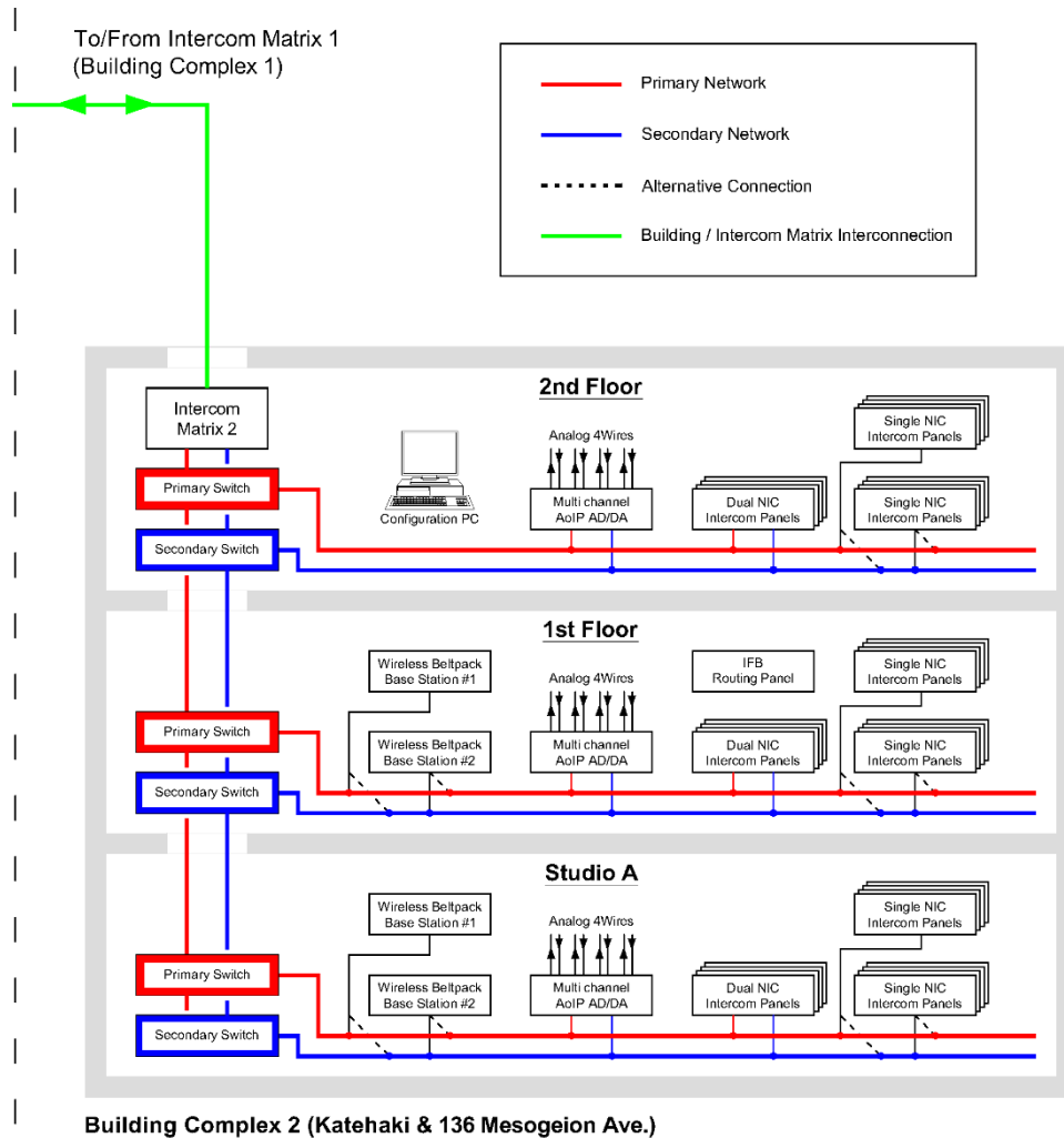
Σχήμα 2: Σχηματικό διάγραμμα συστήματος στο κτηριακό συγκρότημα της Κατεχάκη
