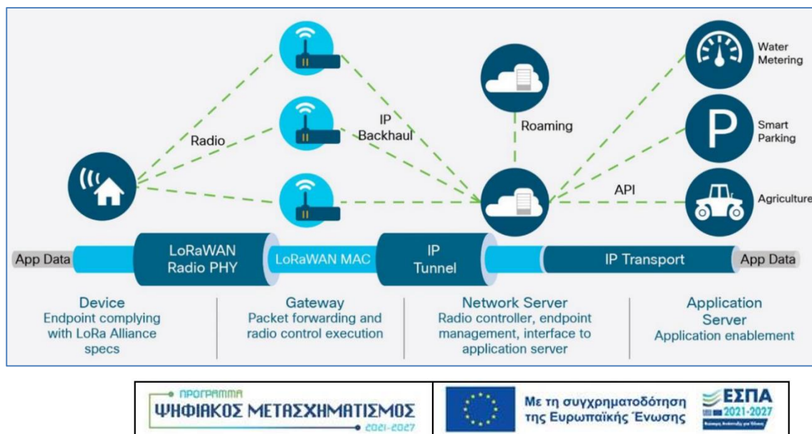
Εικόνα 1 Αρχιτεκτονική Δικτύου LoRaWAN
