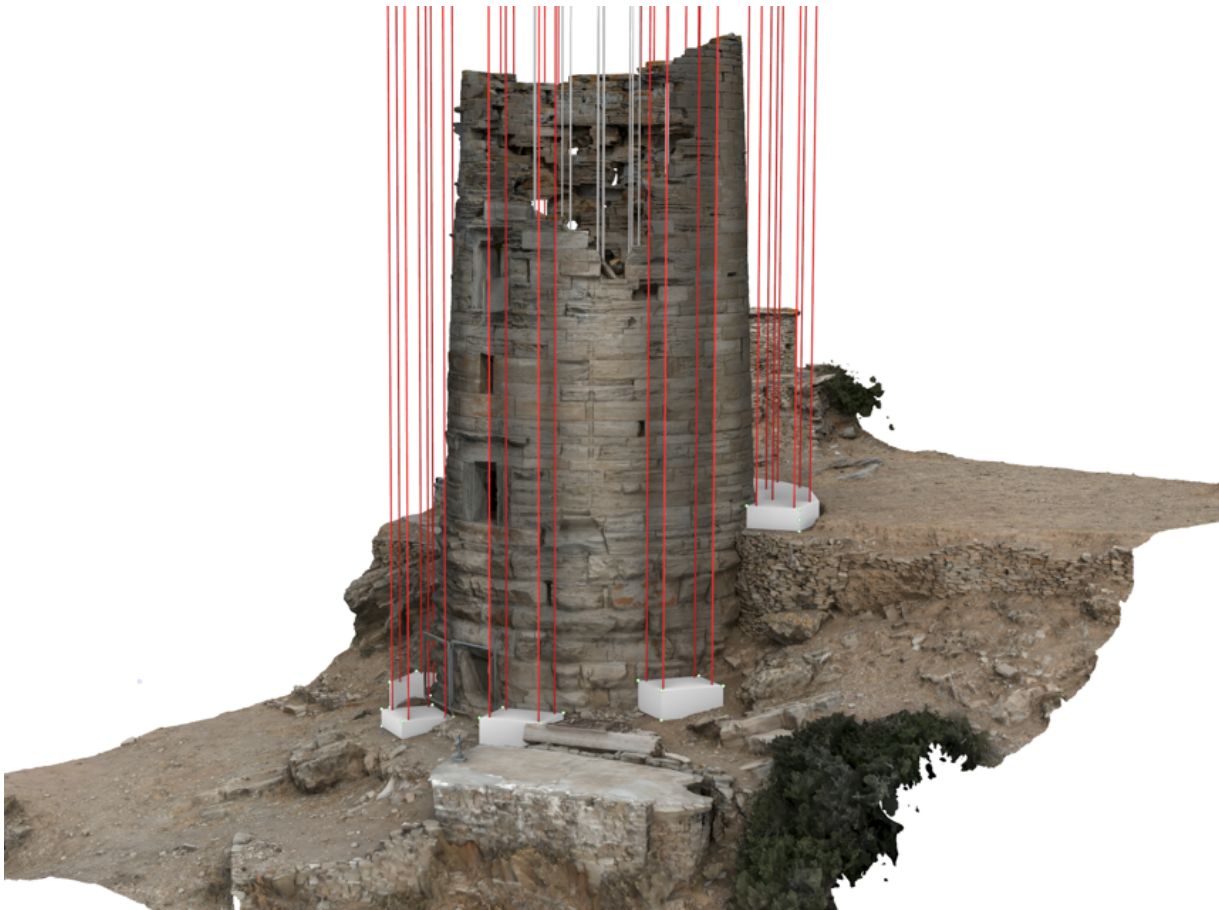
Εικόνα 2 Ο πύργος με τις βάσεις και τις θέσεις τοποθέτησης των εξωτερικών πύργων του ικριώματος από νότιοανατολικά.
