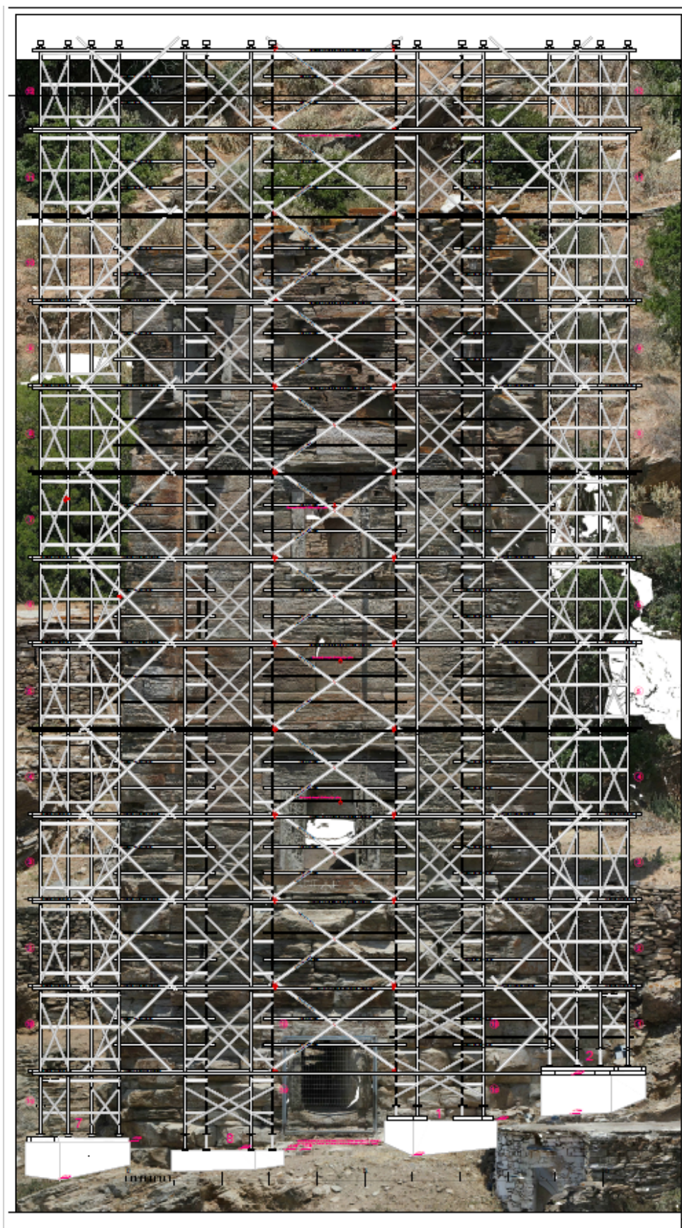
Εικόνα 6 Νότια όψη (Γερ. Θωμάς 2022)
