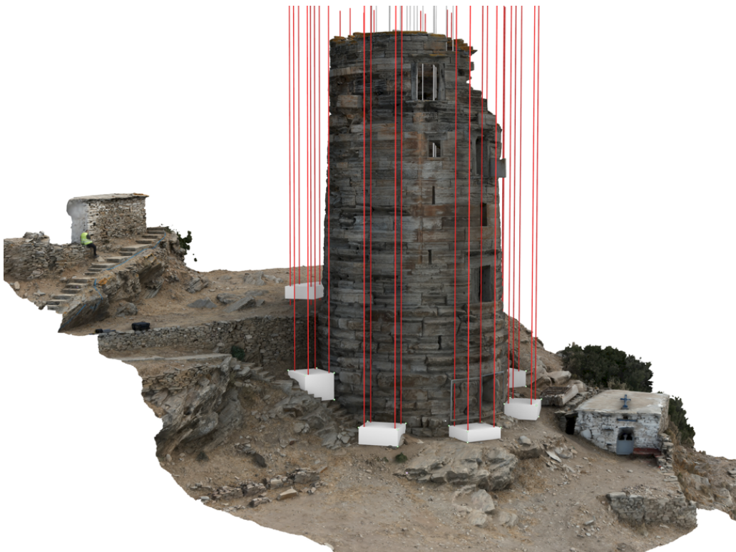
Εικόνα 1 Ο πύργος με τις βάσεις και τις θέσεις τοποθέτησης των εξωτερικών πύργων του ικριώματος από νοτιοδυτικά.
