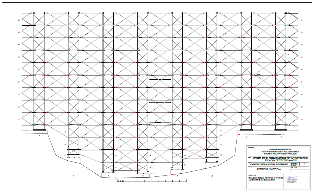
Εικόνα 7 Εξωτερικό ανάπτυγμα ικριώματος (Γερ. Θωμάς 2022)
