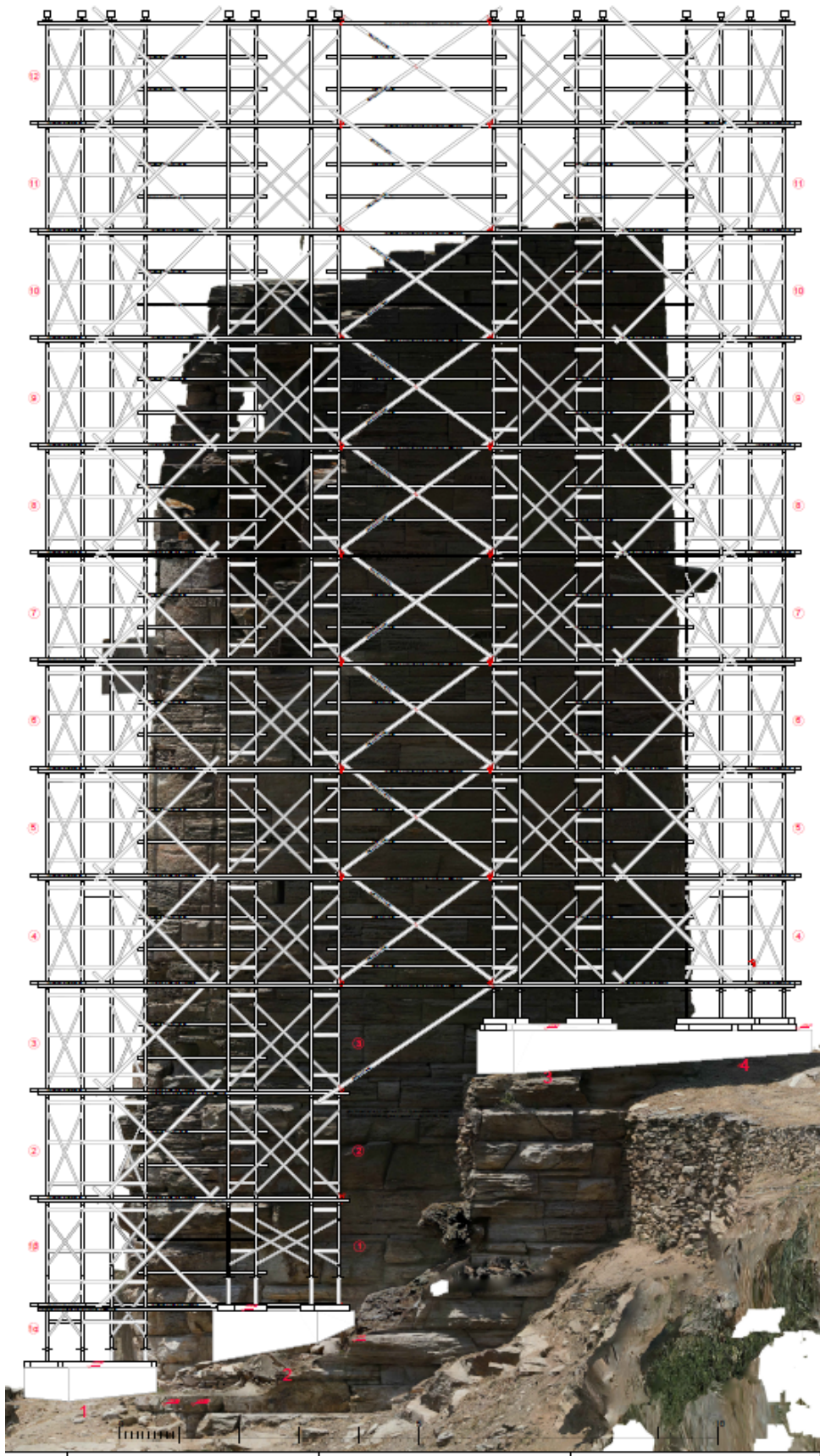
Εικόνα 4 Ανατολική όψη (Γερ. Θωμάς 2022)
