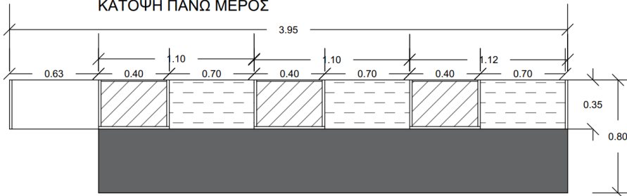
ΚΑΤΟΨΗ ΠΑΝΩ ΜΕΡΟΣ
