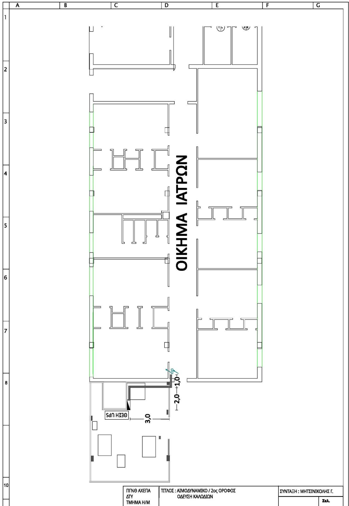
Σχέδιο 8 / Τμήμα 2 : Όδευση καλωδίων / Αιμοδυναμικό Εργαστήριο / 1ος όροφος
