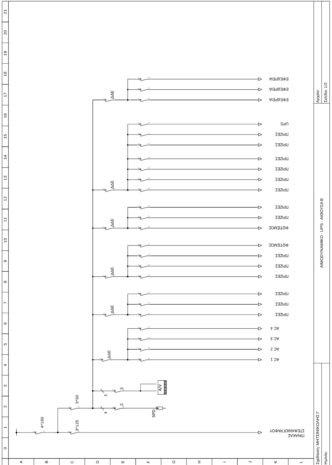
Σχέδιο 5 / Τμήμα 2 : Υφιστάμενος πίνακας αίδουσας Β' / Αιμοδυναμικό Εργαστήριο
