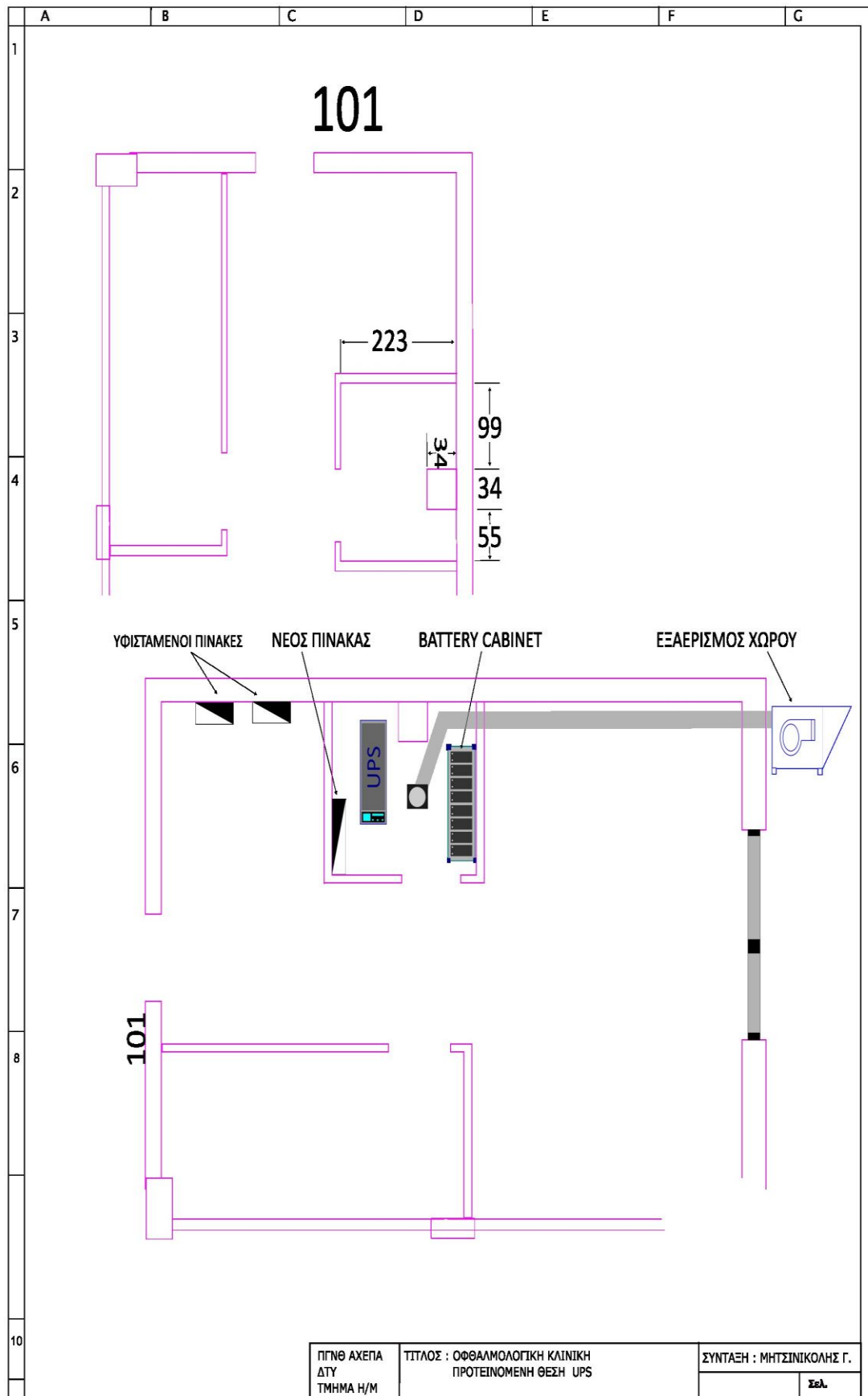
Σχέδιο 3 / Τμήμα 1 : Οφθαλμολογική κλινική – Προτεινόμενη θέση UPS
