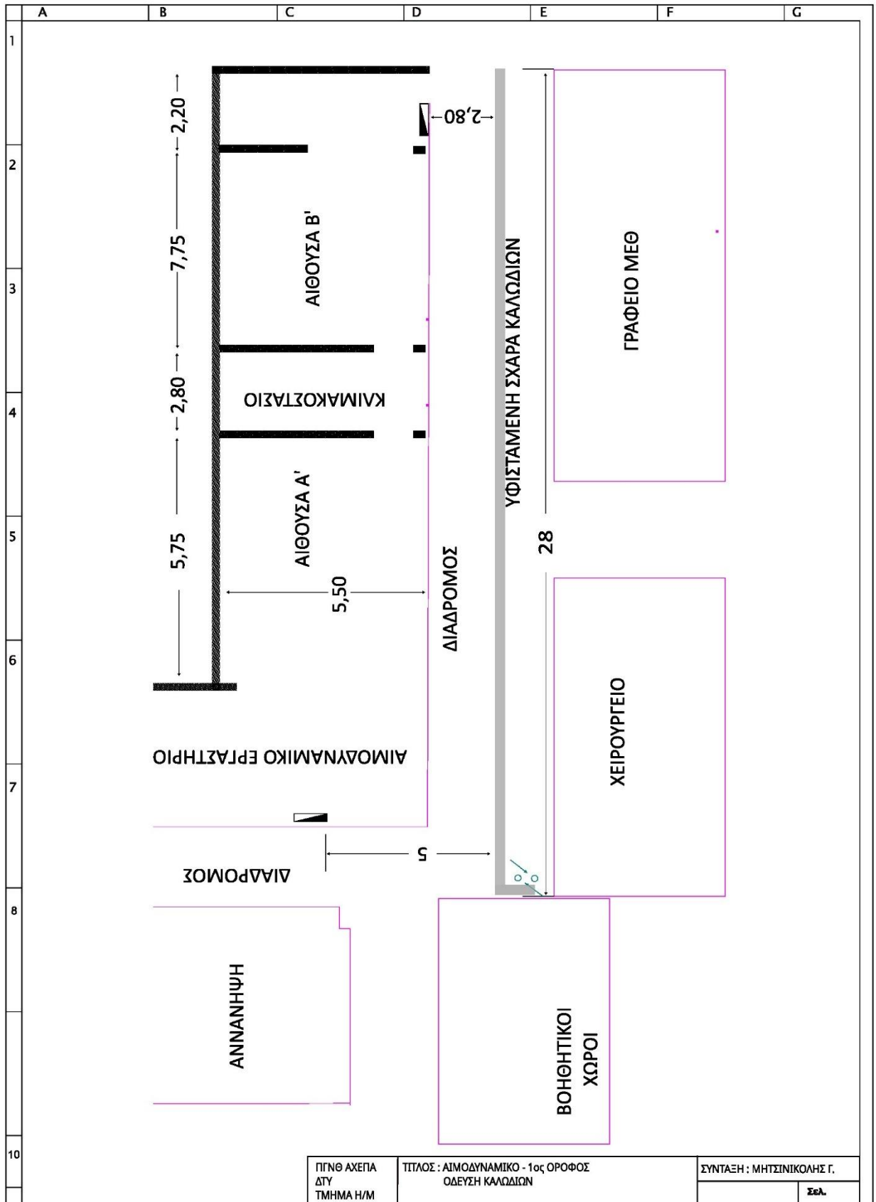
Σχέδιο 7 / Τμήμα 2 : Όδευση καλωδίων / Αιμοδυναμικό Εργαστήριο / 1ος όροφος
