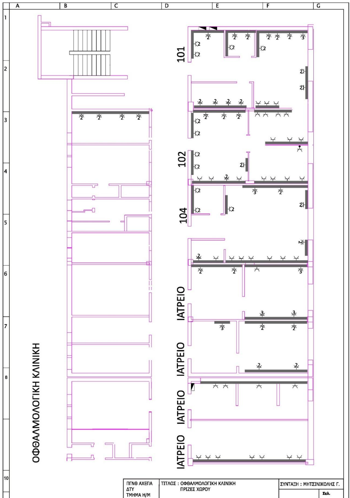
Σχέδιο 4 / Τμήμα 1 : Οφθαλμολογική κλινική – Πρίζες χώρους
