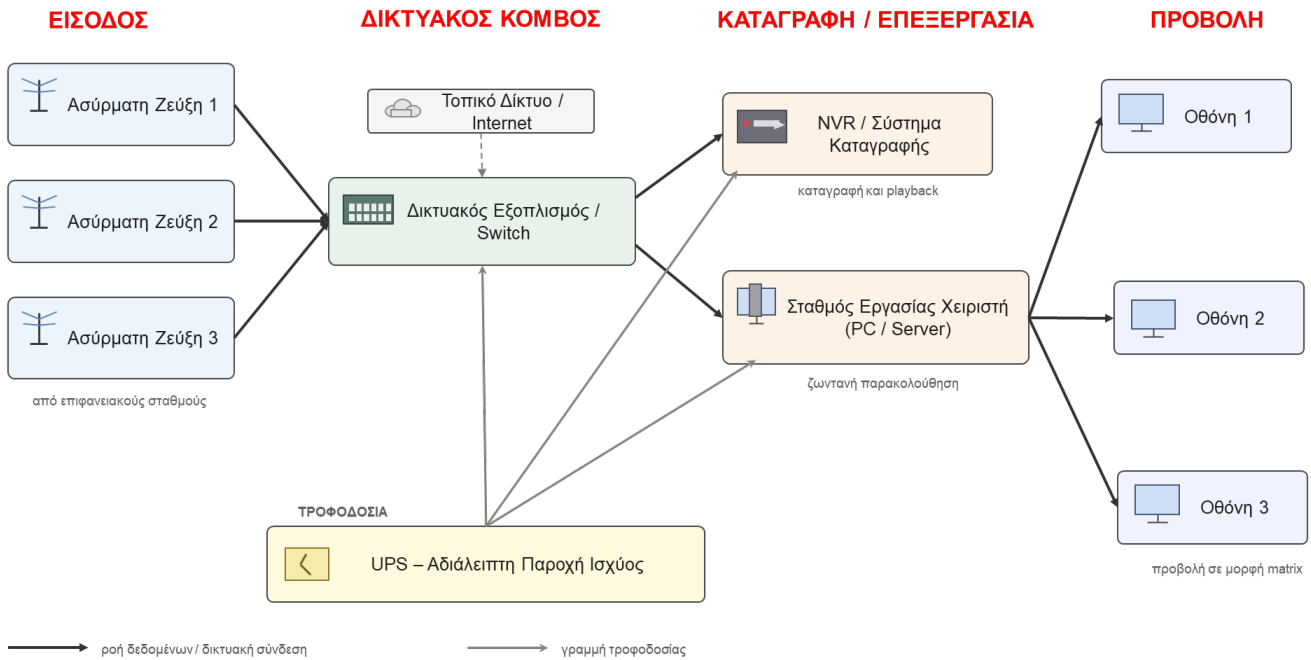
Σχήμα: Συνοπτική Αναπαράσταση Λειτουργίας Κέντρου Επιτήρησης - Προβολής - Παρουσίασης
