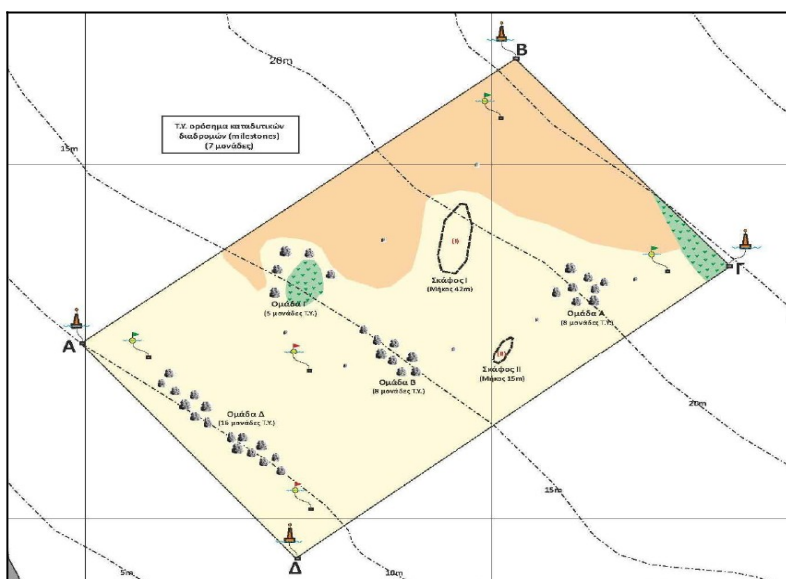
Σχήμα: Γενική Διάταξη Καταδυτικού Πάρκου
