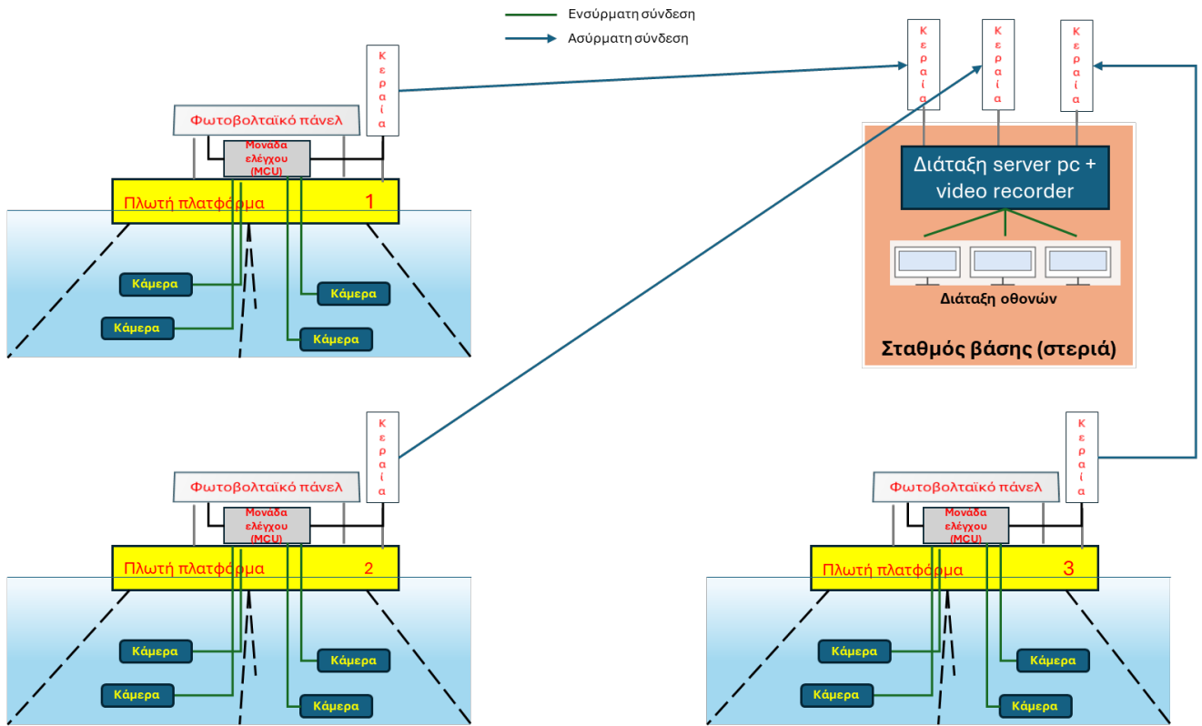
Σχήμα: Συνοπτική Αναπαράσταση Αρχιτεκτονικής του Συστήματος Παρακολούθησης του Καταδυτικού Πάρκου
