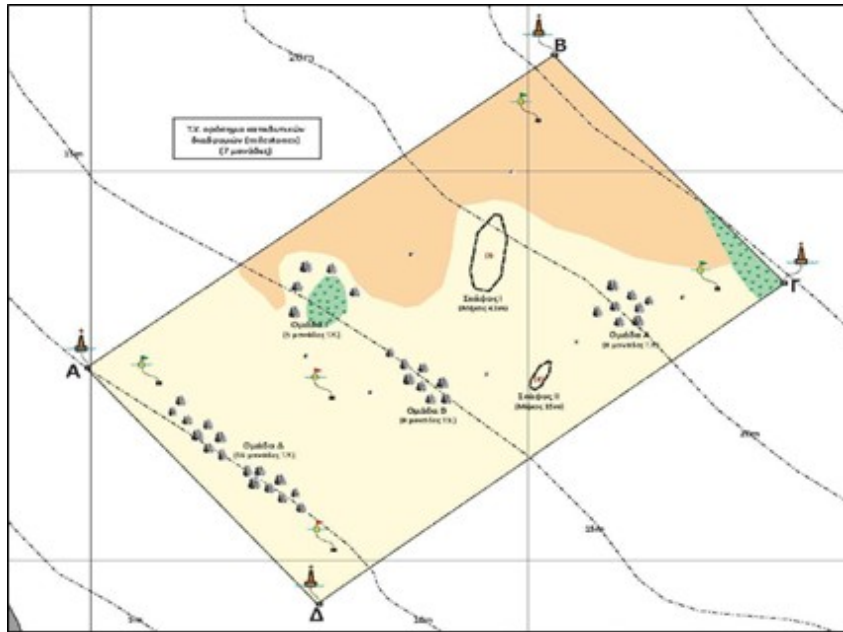
Σχήμα : Γενική Διάταξη Καταδυτικού Πάρκου
