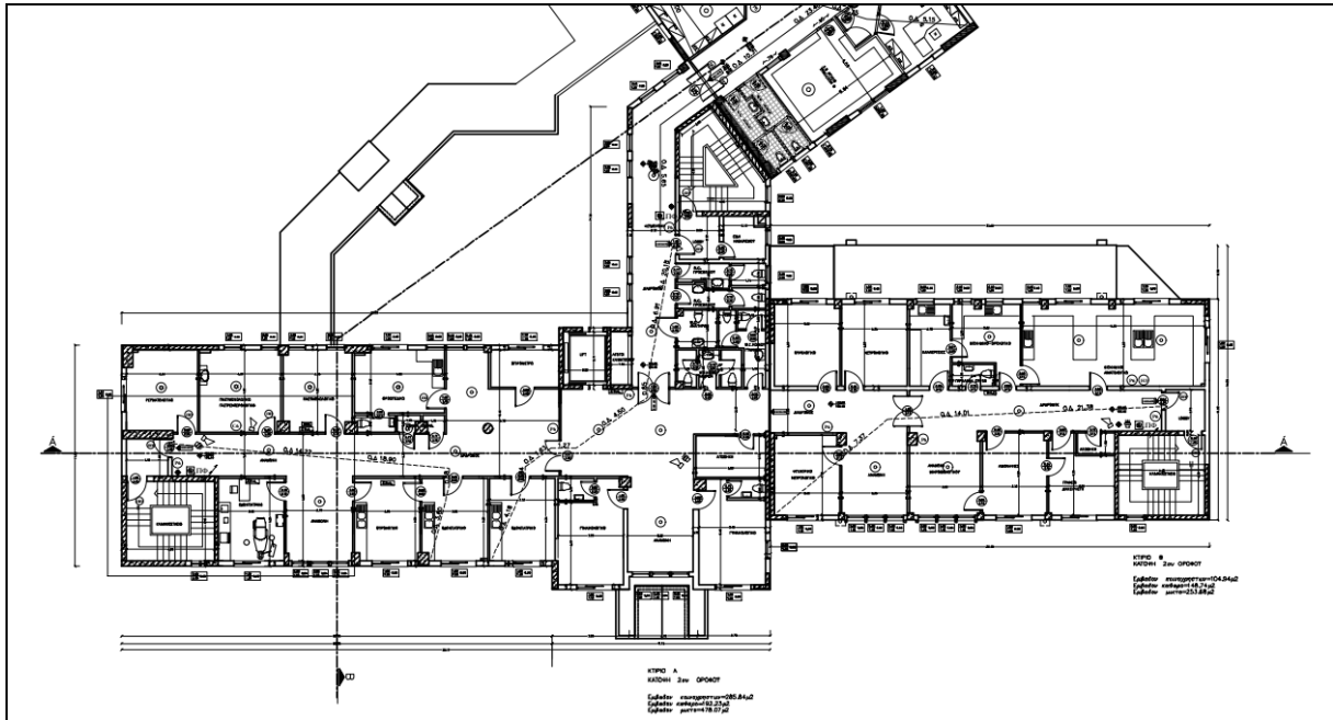
Εικόνα 3. Κάτοψη 2 ου ορόφου Κ.Υ. Τούμπας
