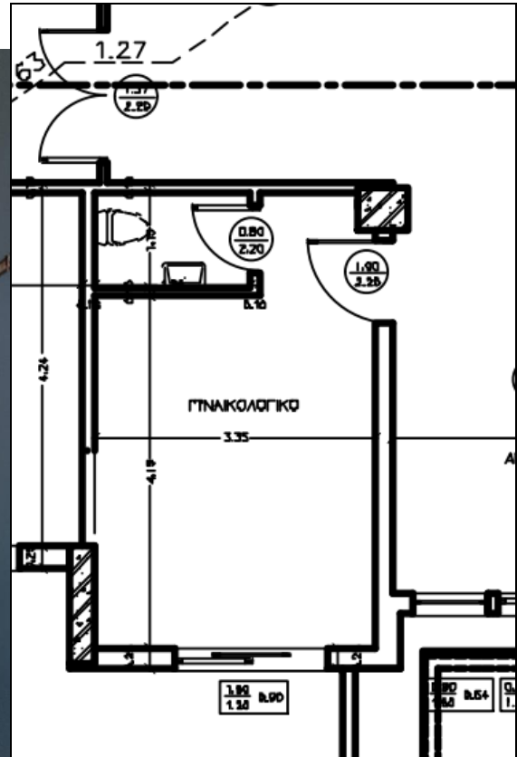
Εικόνα 6. Κάτοψη WC του 2 ου ορόφου
