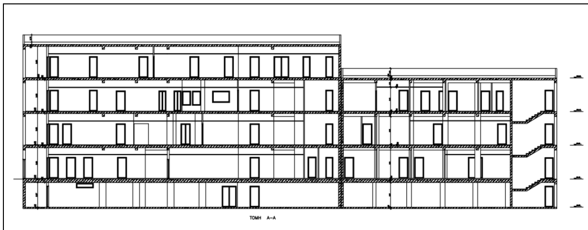
Εικόνα 7. Τομή Α-Α Κ.Υ. Τούμπας
