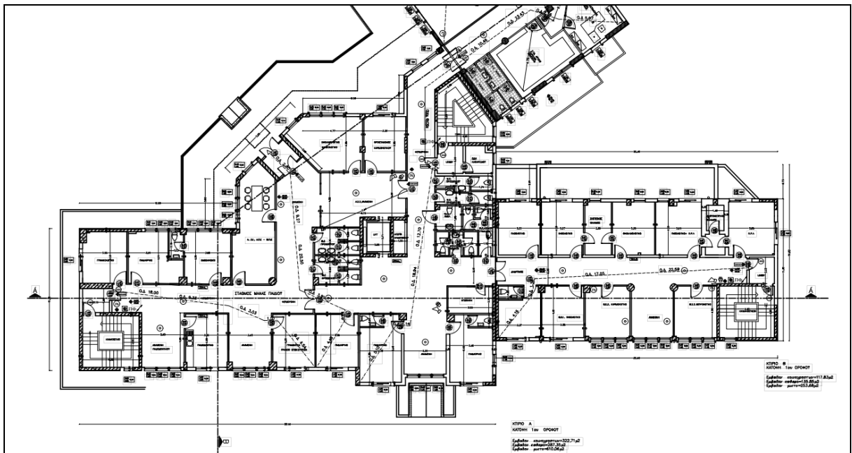
Εικόνα 2. Κάτοψη 1 ου ορόφου Κ.Υ. Τούμπας
