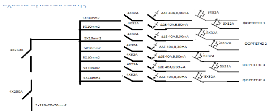
Σχήμα 3: Μονογραμμικό σχέδιο εγκατάστασης
