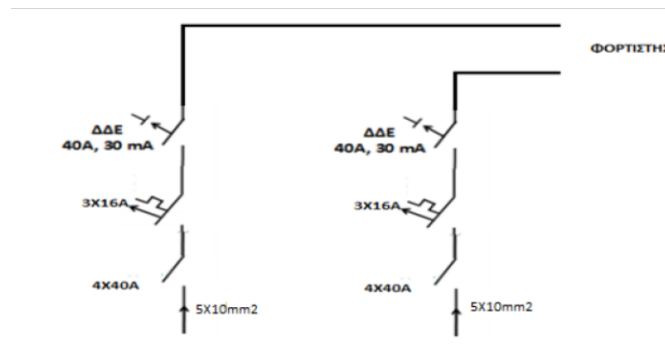
Σχήμα 1: Μονογραμμικό σχέδιο εγκατάστασης
