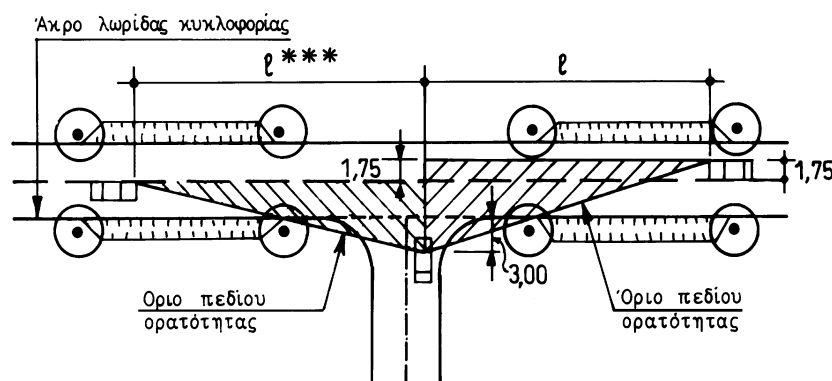
Σχήμα 3: Ορατότητα για εκκίνηση οχήματος από δευτερεύουσα οδό για είσοδο σε κύρια οδό. Το μήκος L = 200\mu
