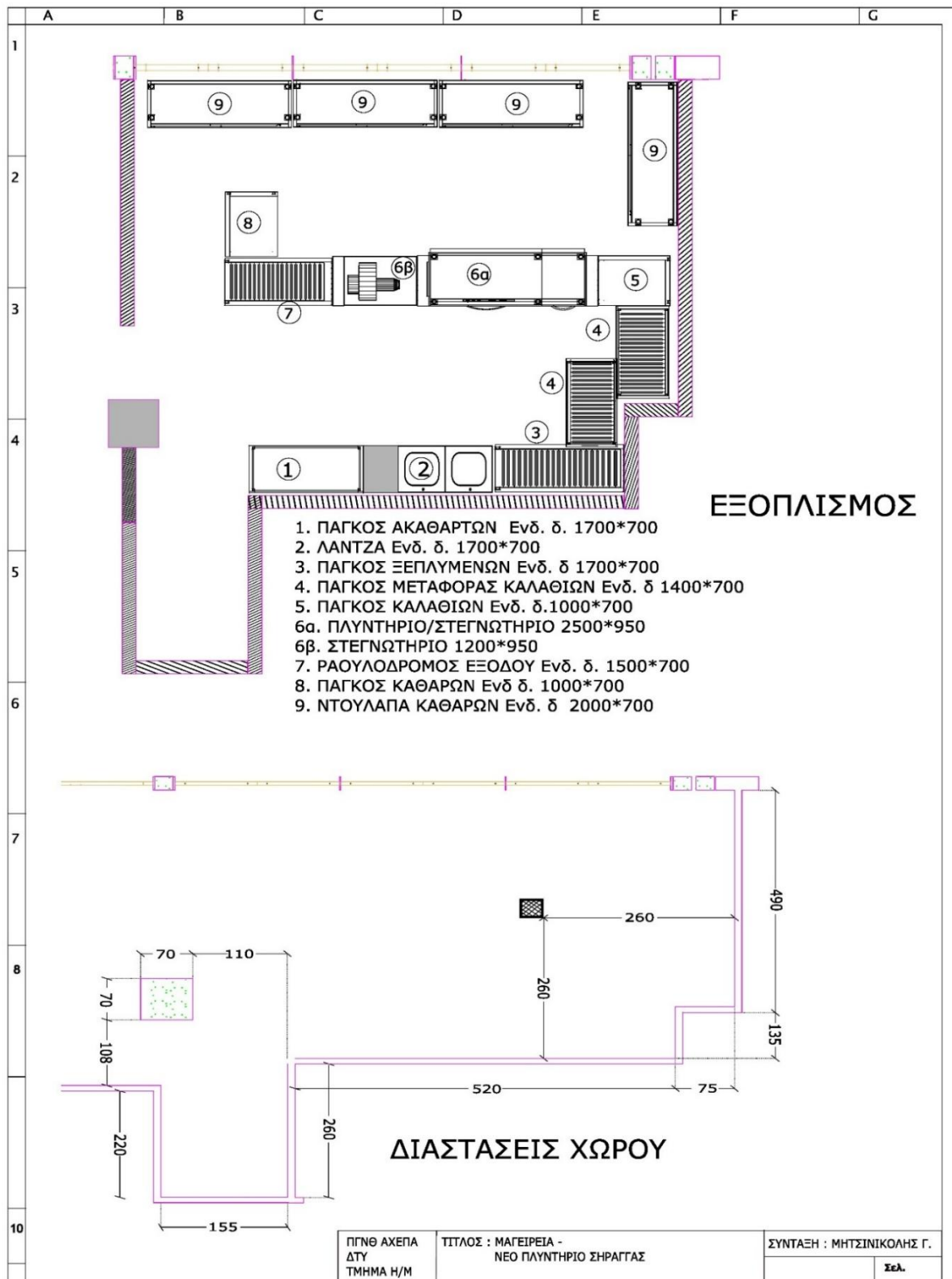
Σχέδιο 3.3: Συνοδος Εξοπλισμός χώρου πλυντηρίου τούνελ.
