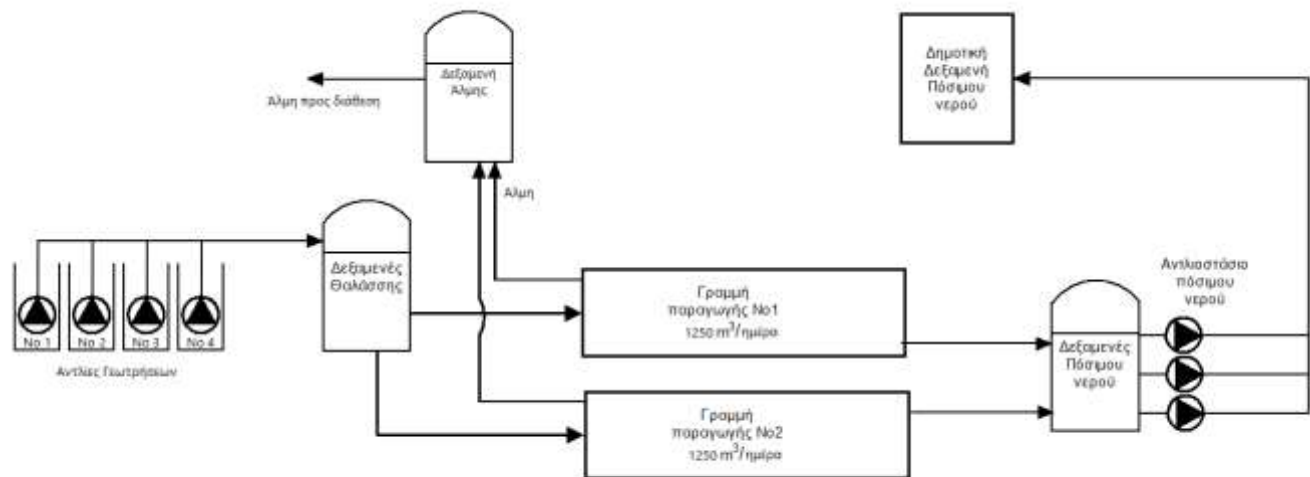
Σχήμα 1 : Διάγραμμα σταδίων της μονάδας αφαλάτωσης 2.500 m³/ημέρα
