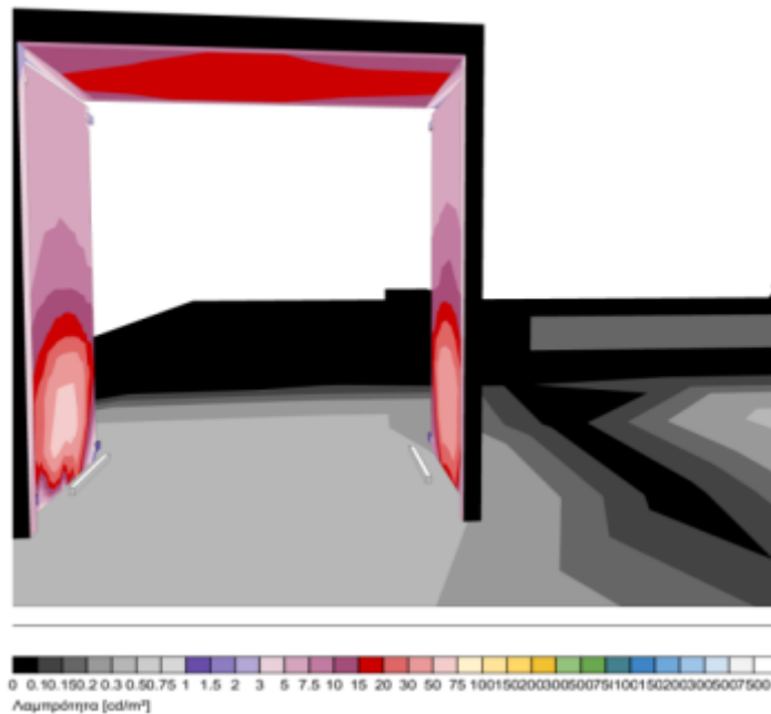
Εικόνα Β.2.16.στ Ενδεικτική 3D Κατανομή λαμπρότητας στο εσωτερικό της θύρας (φ/σ ενδεικτικού τύπου)
