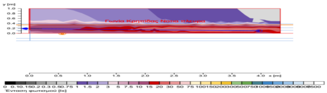
Εικόνα Β.2.20.δ Επισκόπηση αποτελεσμάτων έντασης φωτισμού με ψευδοχρώματα (Νότια πλευρά κρητίδας)
