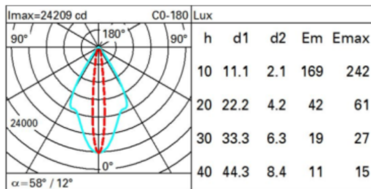
Εικόνα Β.2.6.α Ενδεικτικό πολικό διάγραμμα Φωτεινής Έντασης (φ/σ ενδεικτικού τύπου)
