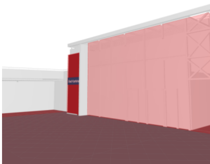
Εικόνα Β.2.11.β Ενδεικτική τοποθέτηση του γραμμικού ενδοδαπέδιου φωτιστικού μπροστά από το μπάρερ
