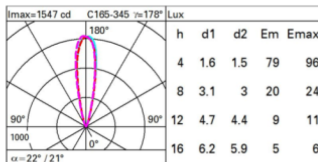
Εικόνα Β.2.17.α Ενδεικτικό πολικό διάγραμμα Φωτεινής Έντασης (φ/σ ενδεικτικού τύπου)
