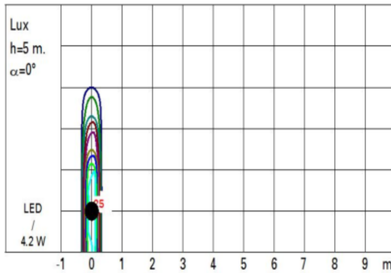
Εικόνα Β.2.4.γ Ενδεικτική isoluminance κατανομή Φωτεινής Έντασης (φ/σ ενδεικτικού τύπου)
