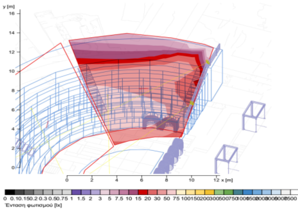
Εικόνα Β.2.6.ζ Επισκόπηση αποτελεσμάτων έντασης φωτισμού με ψευδοχρώματα (δεξιά πτέρυγα κίλου)
