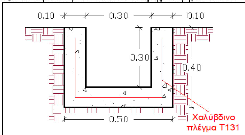
Διατομή αύλακα που θα κατασκευαστεί στο ανατολικό όριο του αγροτεμαχίου
