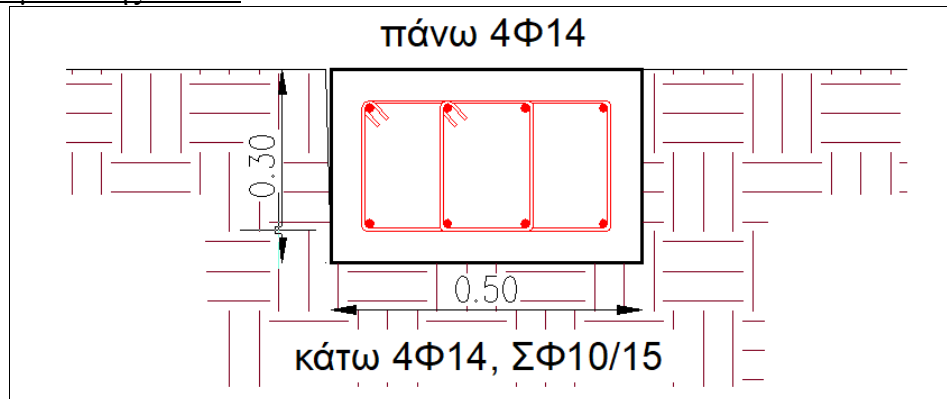
Διάταξη θεμελίου αργολιθοδομών πλάτους 0.50m
