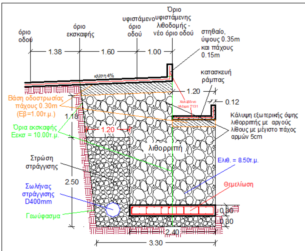
Γενική διάταξη (τομή) κατασκευής λιθορριπής και στραγγιστηρίου στη Χ.Θ. 0+225
