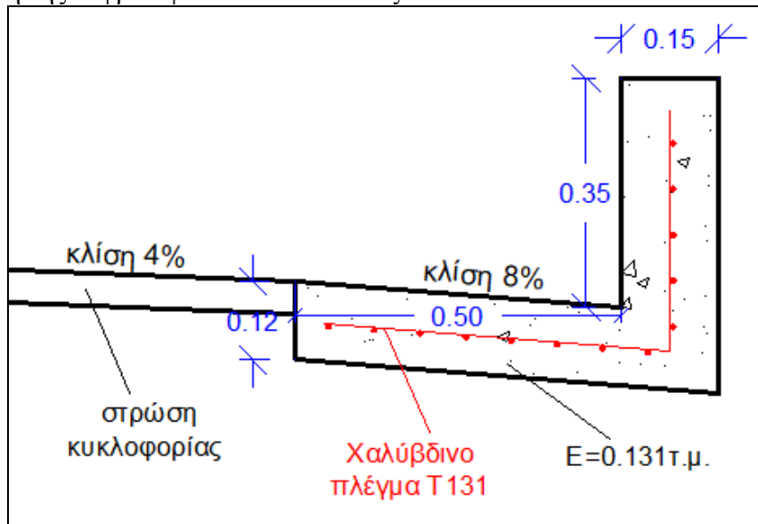
Διατομή επενδεδυμένης τριγωνικής τάφρου απορροής ομβρίων
