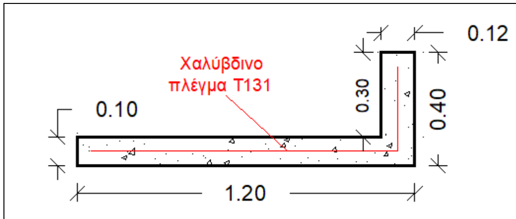
Διατομή επένδυσης ράμπας με οπλισμένο σκυρόδεμα
