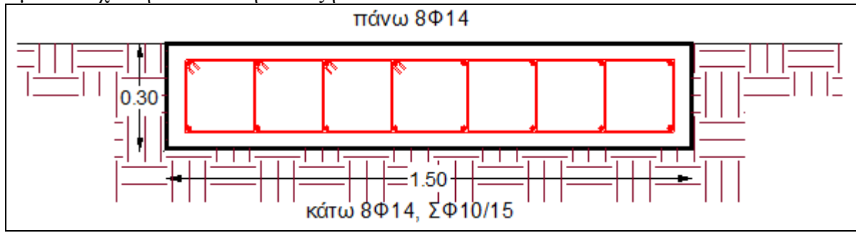
Διάταξη θεμελίου αργολιθοδομής με πλάτος θεμελίου 1.50m
