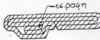
ΤΟΜΗ Β-Β
