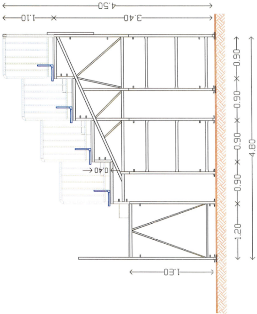
ΕΝΔΕΙΚΤΙΚΗ ΤΟΜΗ
