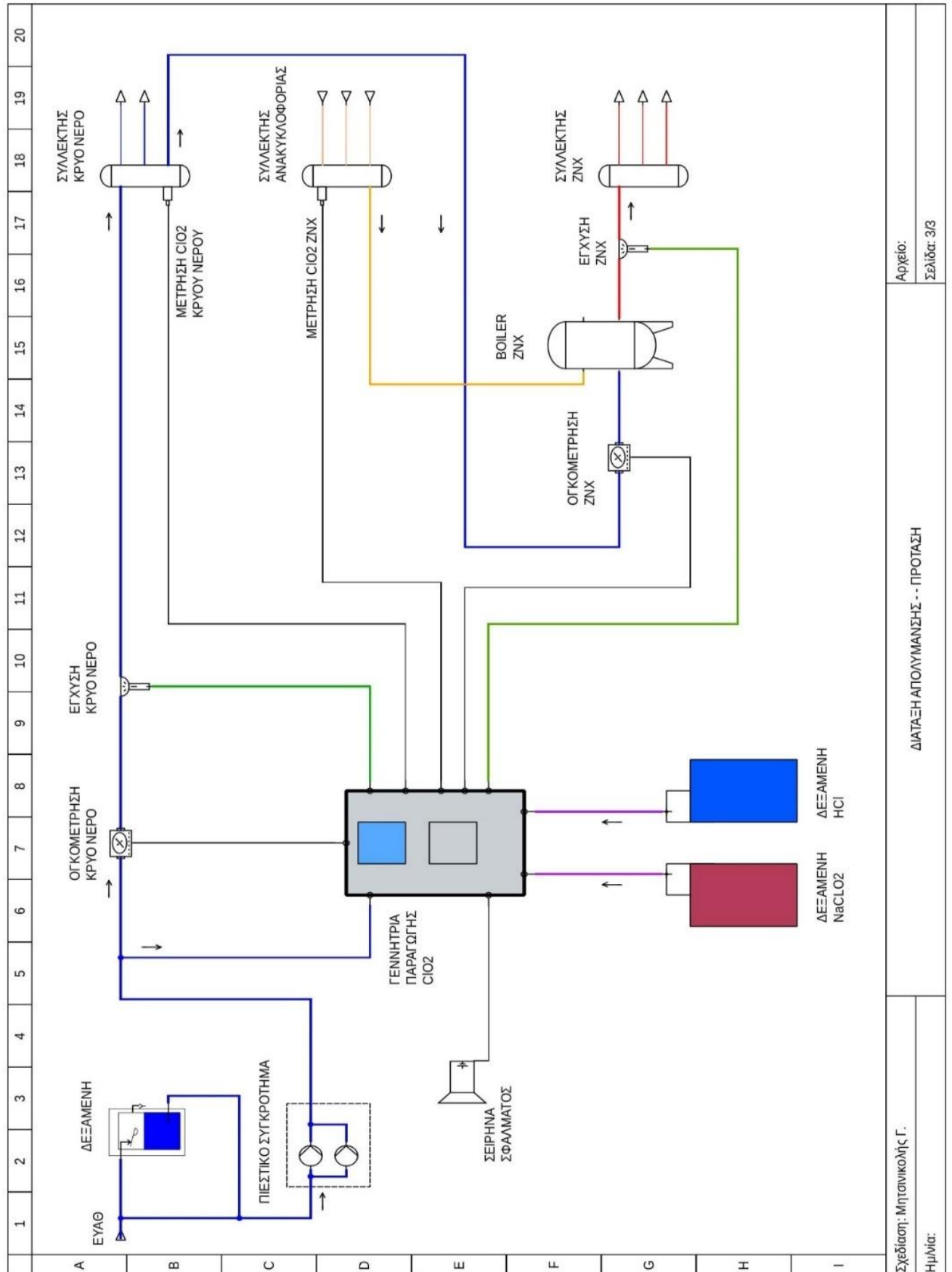
Σχέδιο 2: Πρόταση διάταξης απολύμανσης με ClO 2 για κάθε κτηριακό συγκρότημα
