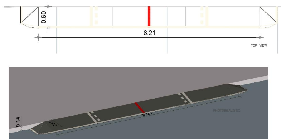
ΣΧ.6α ΡΑΜΠΑ ΕΙΣΟΔΟΥ ΑΘΛΗΤΩΝ/ΑΥΤ. ΚΑΛΛΙΜΑΡΜΑΡΟ
