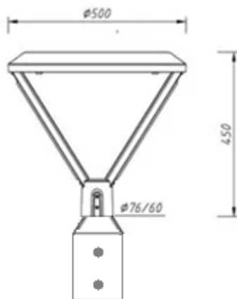
Εικόνα 7. Ενδεικτική απεικόνιση επιθυμητής μορφής φωτιστικού με ανταπτορα.
