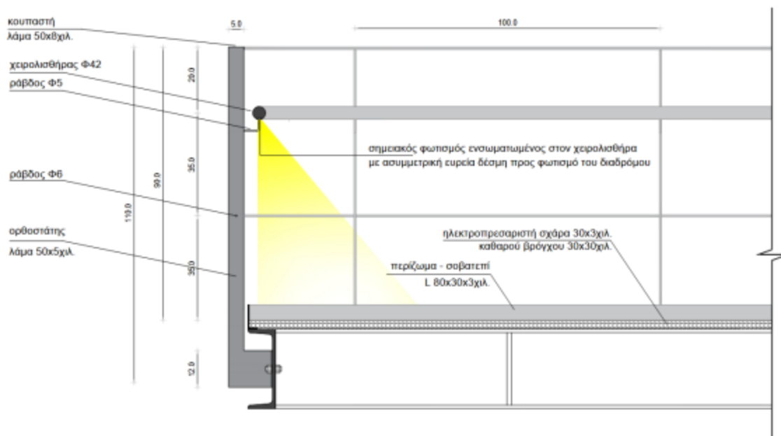
Σχ.3 Πρόταση φωτισμού κιγκλιδώματος
