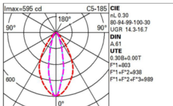
Εικόνα Β.2.13 Ενδεικτικό πολικό διάγραμμα Φωτεινής Έντασης ( \varphi/\sigma ενδεικτικού τύπου)
