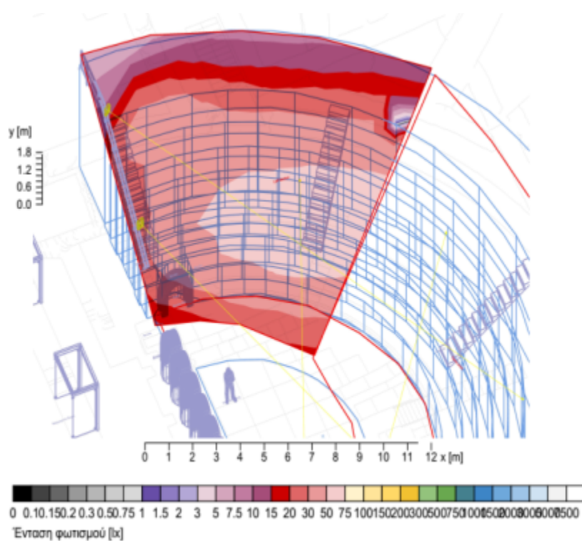
Εικόνα Β.2.6.ε Επισκόπηση αποτελεσμάτων έντασης φωτισμού με ψευδοχρώματα (αριστερή πτέρυγα κοίλου)
