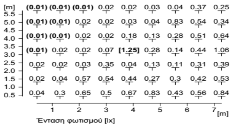
Εικόνα Β.2.20.ζ Επισκόπηση αποτελεσμάτων έντασης φωτισμού σε πίνακα (δάπεδο πλατείας ΝΑ γωνία κρηπίδας)
