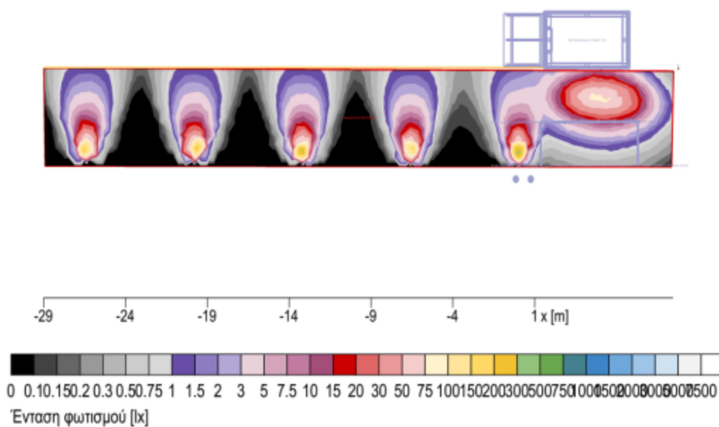
Εικόνα Β.2.3.δ Επισκόπηση αποτελεσμάτων με τη μορφή ψευδοχρωμάτων (φ/σ ενδεικτικού τύπου)
