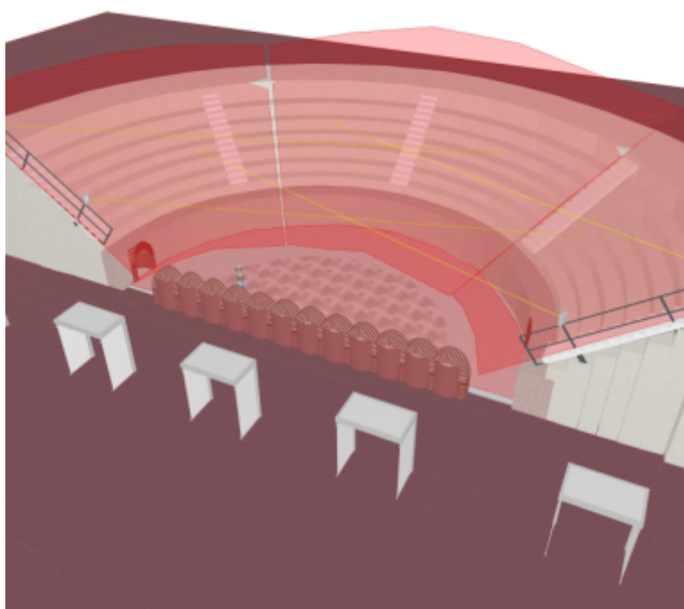
Εικόνα Β.2.6.δ Ενδεικτική τοποθέτηση των φ/σ επί των κιγκλιδωμάτων αμφιπλεύρως στα όρια του κοίλου
