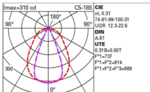
Εικόνα Β.2.15 Ενδεικτικό πολικό διάγραμμα Φωτεινής Έντασης (φ/σ ενδεικτικού τύπου)
