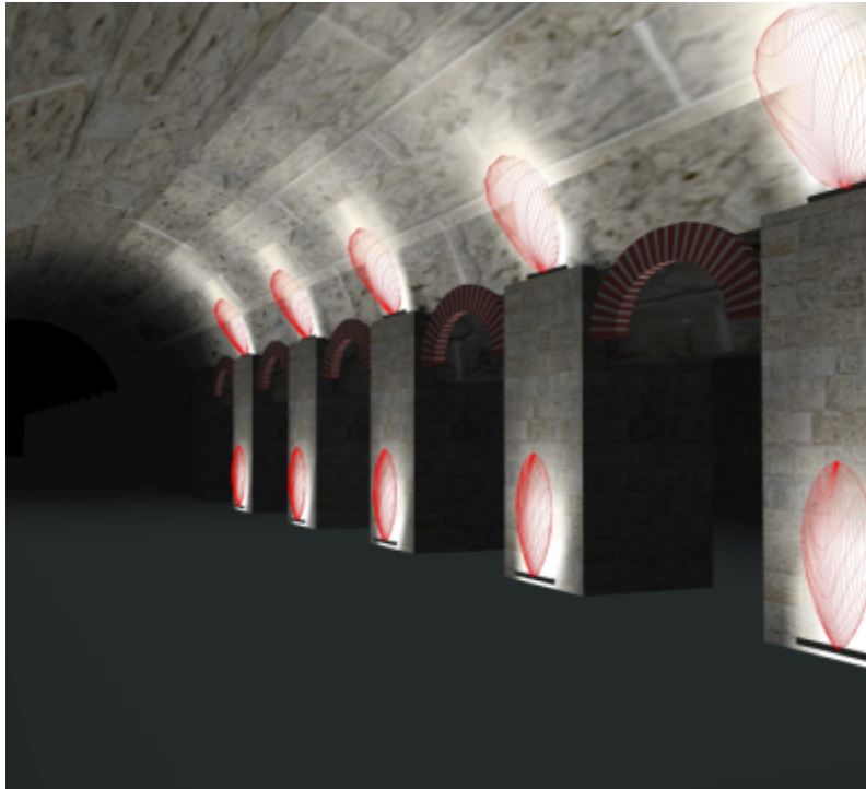
Εικόνα Β.2.12.στ Ενδεικτική 3D Κατανομή λαμπρότητας σε πεσσούς και οροφή θόρειας στοάς (φ/σ ενδεικτικού τύπου)
