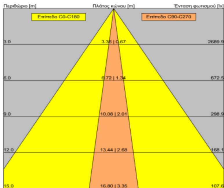
Εικόνα Β.2.6.γ Διάγραμμα κώνου (φ/σ ενδεικτικού τύπου)
