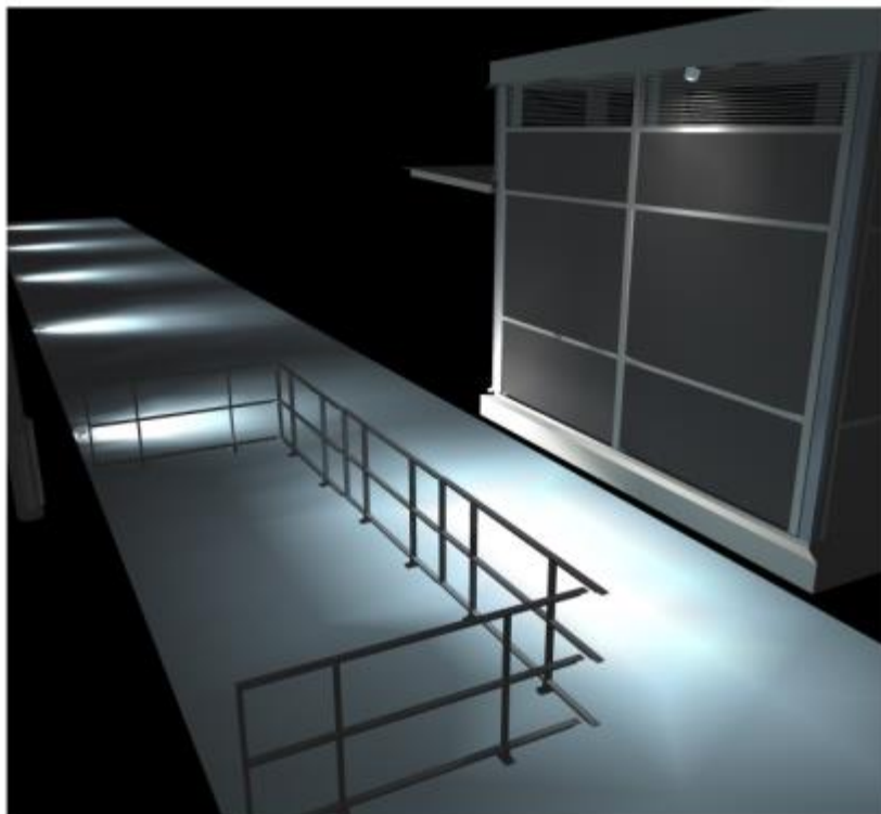
Εικόνα Β.2.3.ε Ενδεικτική 3Δ Κατανομή λαμπρότητας (φ/σ ενδεικτικού τύπου)
