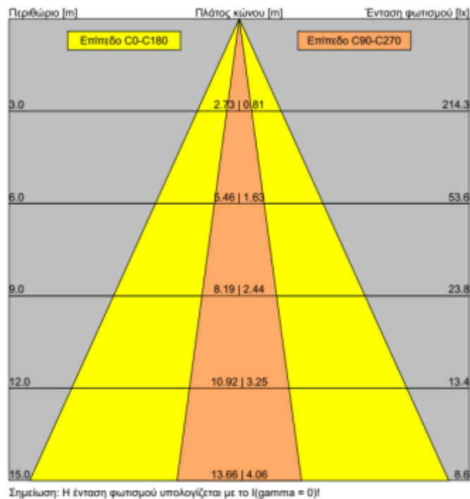
Εικόνα Β.2.3.β Διάγραμμα κώνου (φ/σ ενδεικτικού τύπου)
