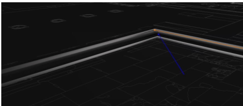
Εικόνα Β.2.20.θ Ενδεικτική 3D Κατανομή λαμπρότητας στη ΝΑ γωνία της κρηπίδας
