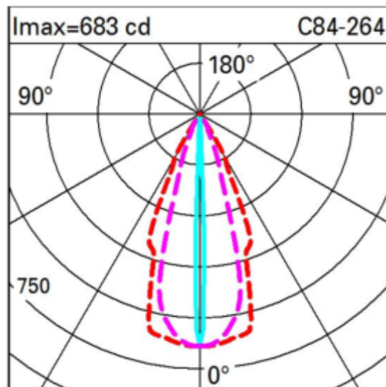
Εικόνα Β.2.4.α Ενδεικτικό πολικό διάγραμμα Φωτεινής Έντασης ( \varphi/\sigma ενδεικτικού τύπου)
