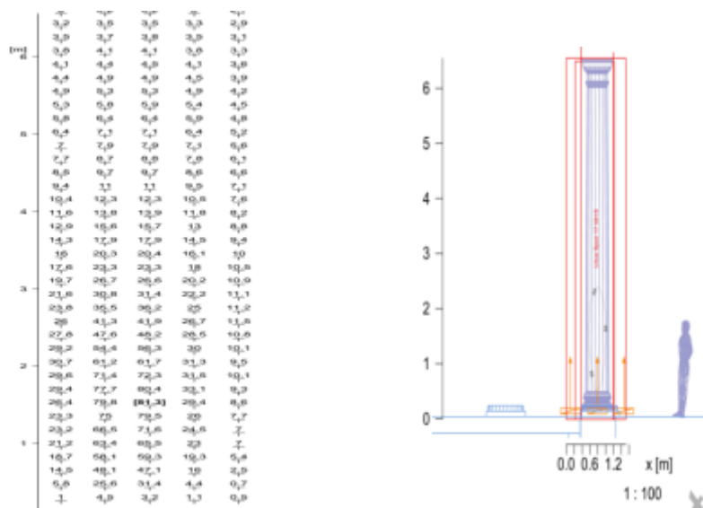
Εικόνα Β.2.18.γ Ενδεικτική τοποθέτηση του σημειακών φωτιστικών περιμετρικά του κίονα
