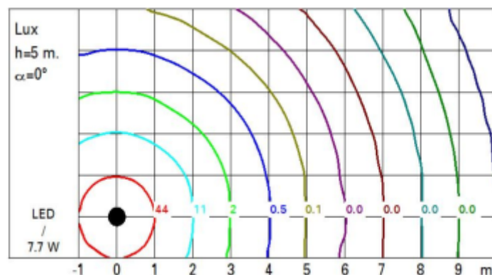
Εικόνα Β.2.10.β Ενδεικτική isolux κατανομή Φωτεινής Έντασης (φ/σ ενδεικτικού τύπου)
