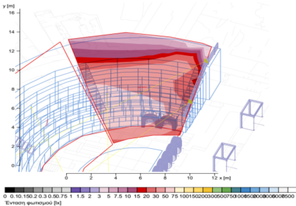
Εικόνα Β.2.6.ζ Επισκόπηση αποτελεσμάτων έντασης φωτισμού με ψευδοχρώματα (δεξιά πτέρυγα κοίλου)
