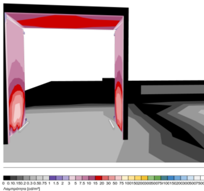
Εικόνα Β.2.16.σ Ενδεικτική 3Δ Κατανομή λαμπρότητας στο εσωτερικό της θύρας (φ/σ ενδεικτικού τύπου)
