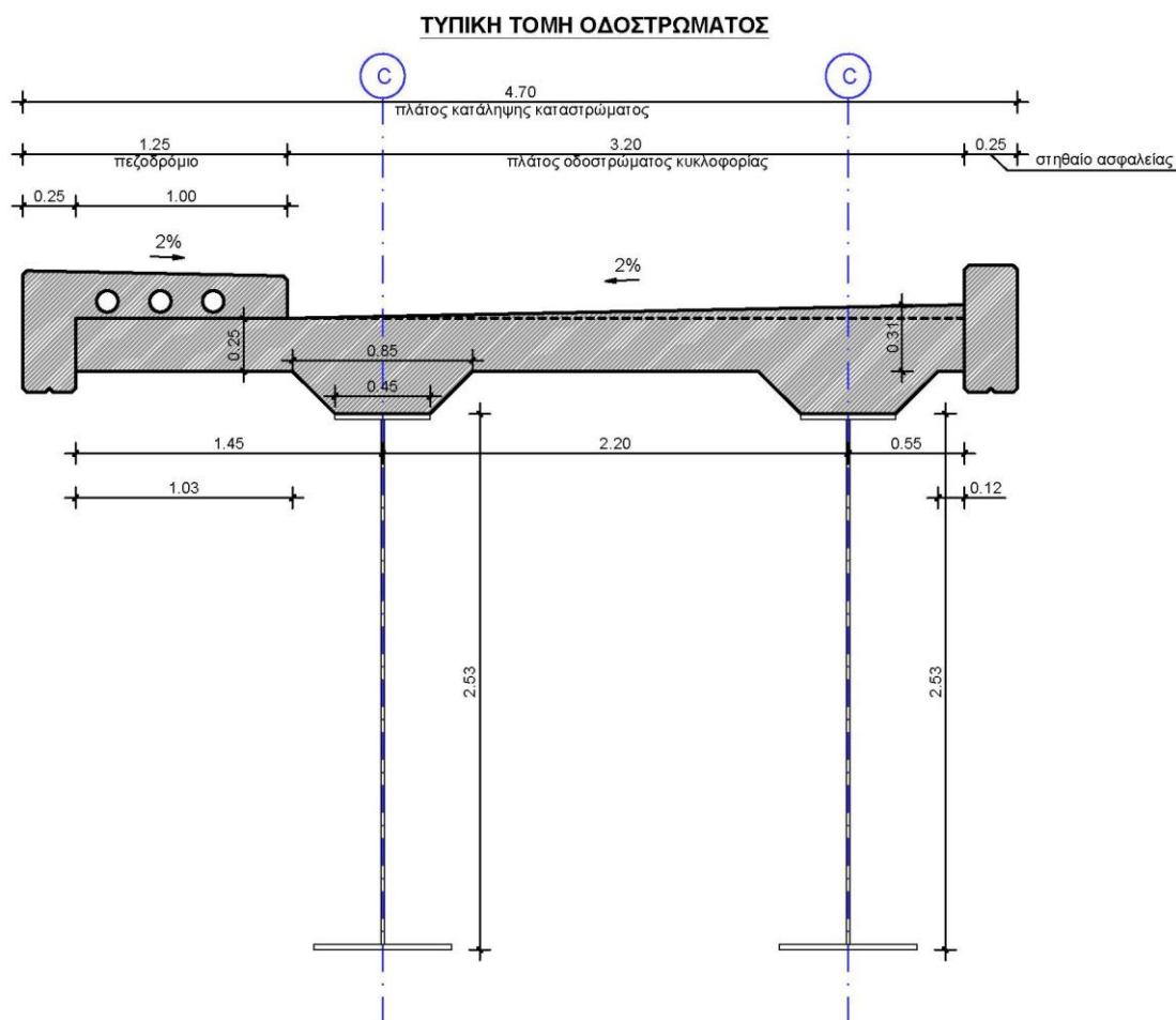
Σχήμα 1. Διατομή φορέα ανωδομής
