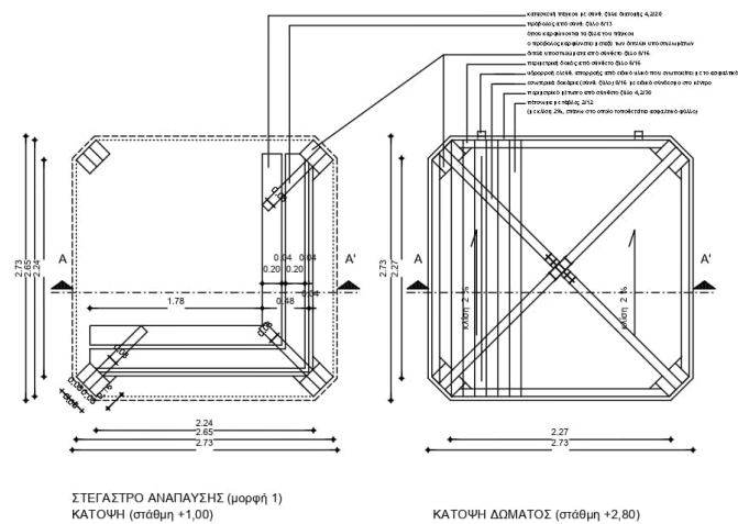
ΚΑΤΟΨΗ ΔΩΜΑΤΟΣ (στάθμη +2,80)
