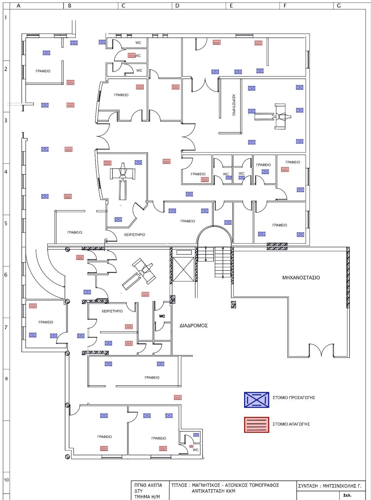
Σχέδιο 2. Στόμια προσαγωγής - απαγωγής
