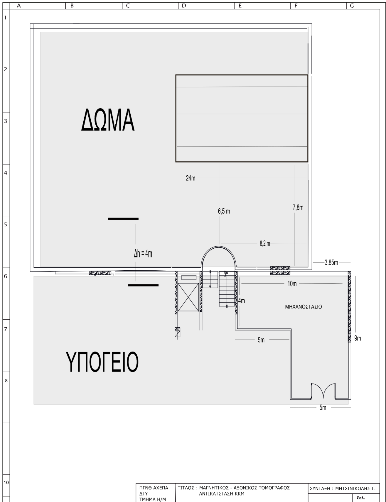
Σχέδιο 3. Δώμα – Διαστάσεις
