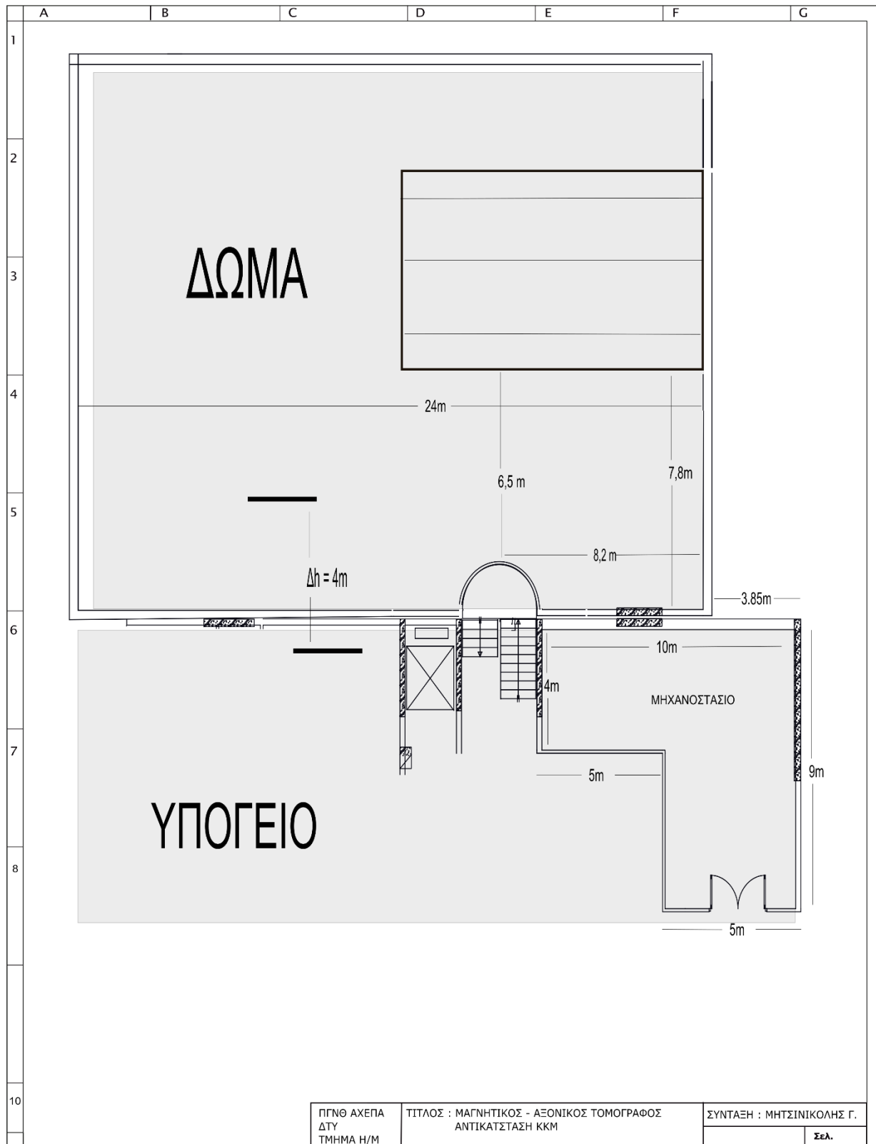
Σχέδιο 3. Δώμα – Διαστάσεις
