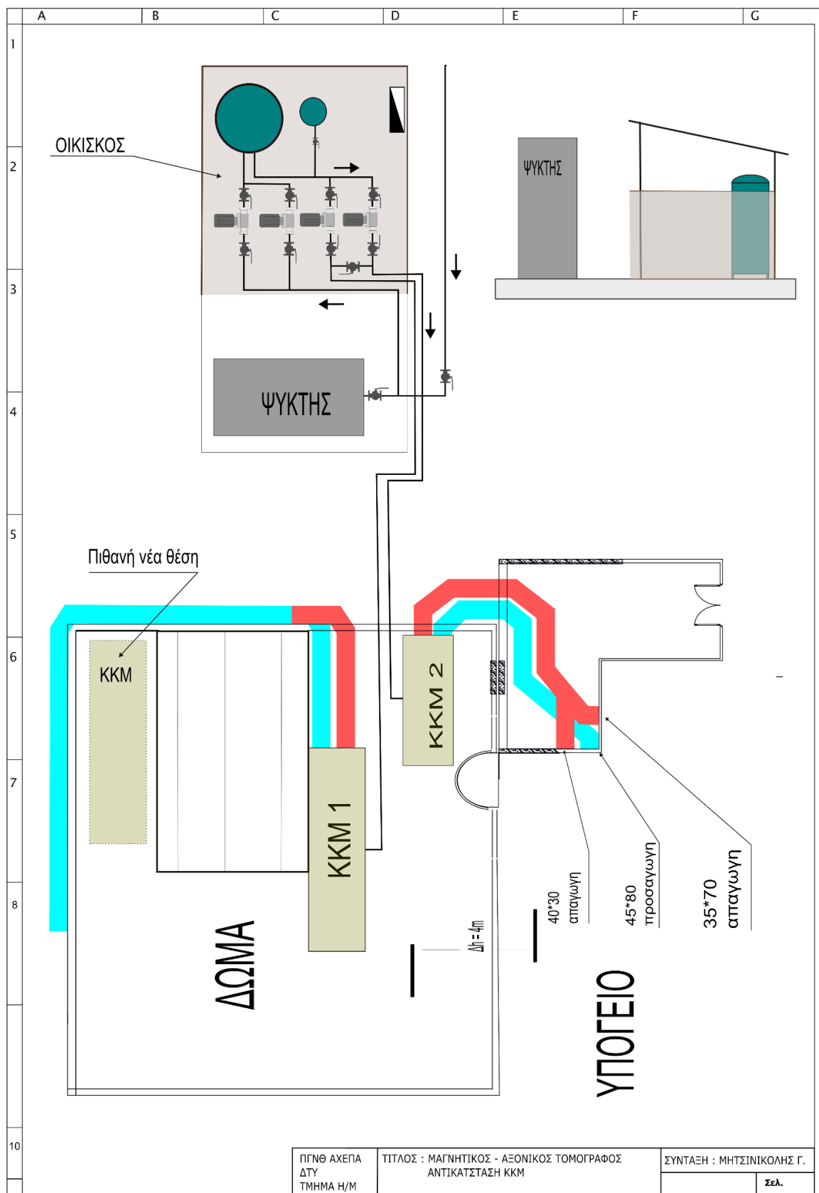
Σχέδιο 4. Ενδεικτική θέση εξοπλισμού - πρόταση
