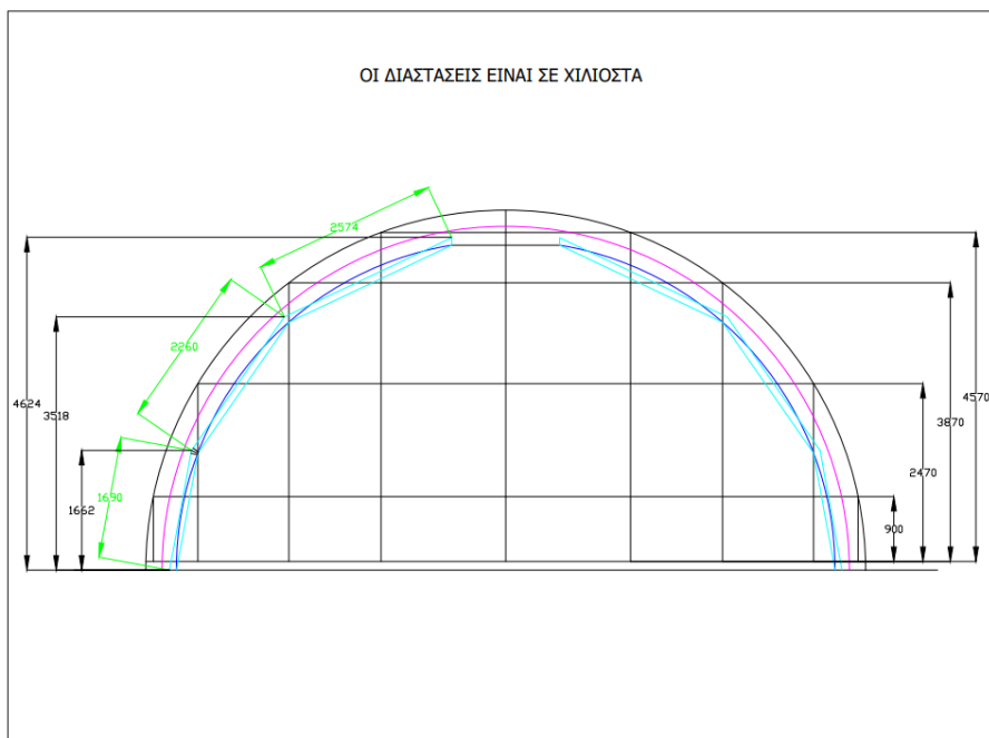
Πίνακας 1. Διαστάσεις igloo
