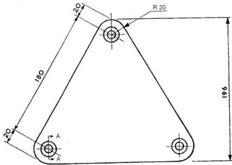
Τρίποδο ηλεκτρόδιο
