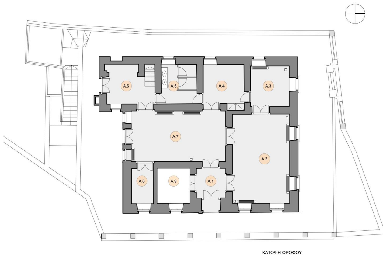
Εικόνα 2: Η κάτοψη του ορόφου, μετά από τις εργασίες αποκατάστασης
