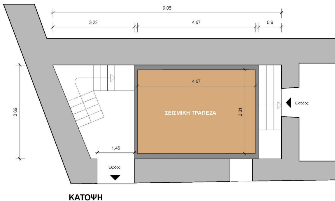
Εικόνα 3: Η κάτοψη του υπογείου, μετά από τις εργασίες αποκατάστασης, με ενδεικτική θέση της Σεισμικής Τράπεζας
