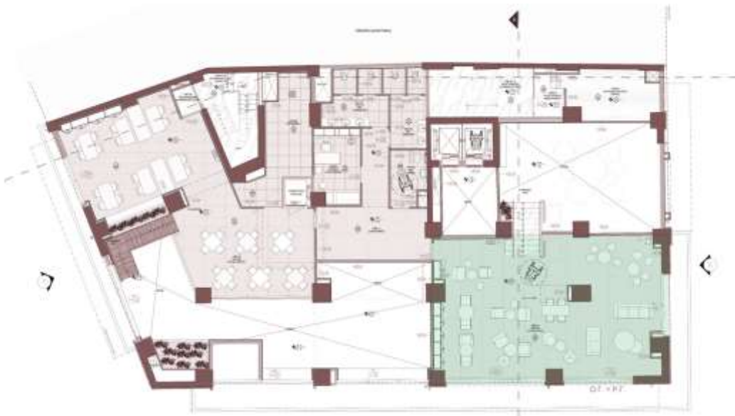
Εικόνα 3: Κάτοψη ημιώροφου (πράσινο: χώρος παιχνιδιού/συνάθροισης)
