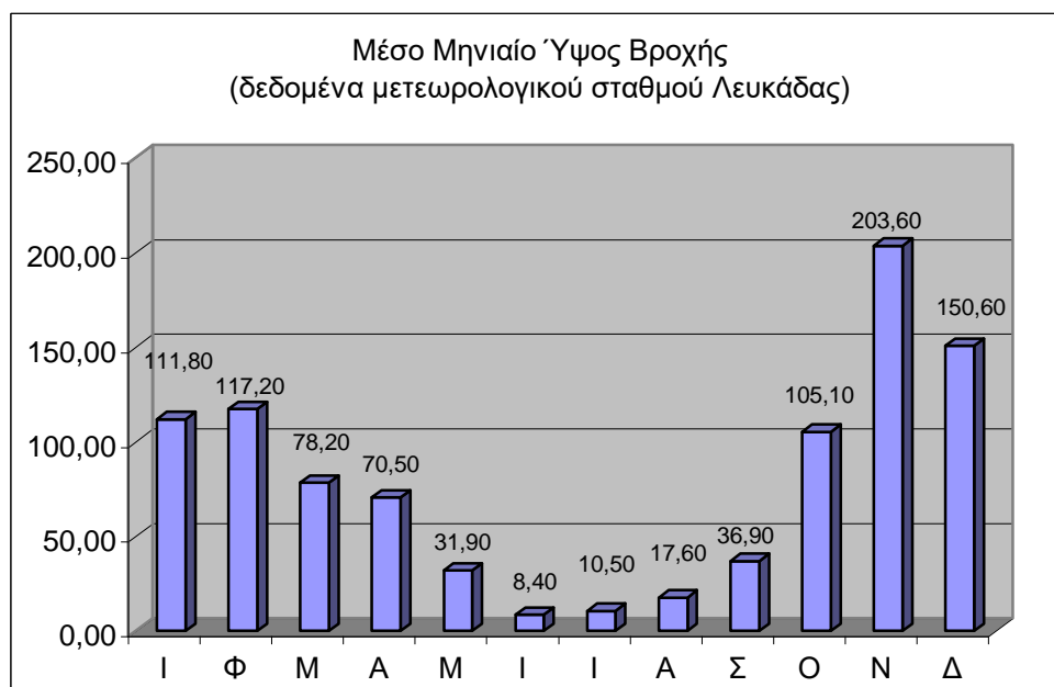
Σχήμα 1.1: Μέσο Μηνιαίο Ύψος Βροχής (δεδομένα μετεωρολογικού σταθμού Λευκάδας)
