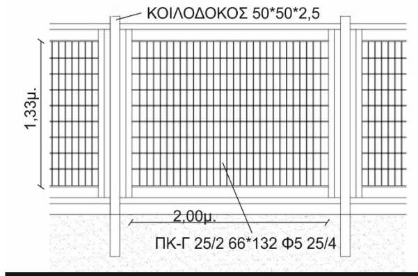
ΣΧΕΔΙΟ ΟΨΗΣ
