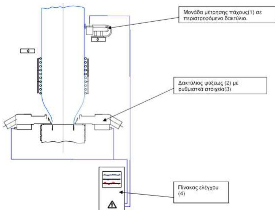
Εικ. 1: Ενδεικτική απεικόνιση ενός δακτυλίου υψηλής απόδοσης με σύστημα μέτρησης σε μονάδα παραγωγής πλαστικού φιλμ μέσω της χρήσης αέρα
