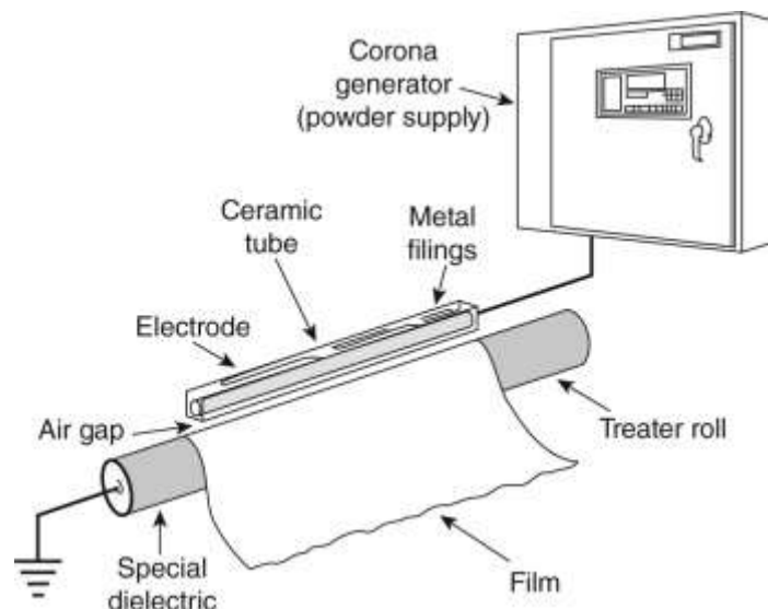
Εικ. 2: Ενδεικτική απεικόνιση λειτουργίας συστήματος επεξεργασίας κορώνας
