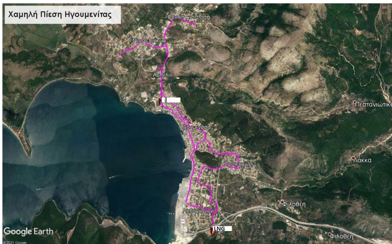
Σχέδιο 5.1. Όδευση δικτύου (main loop) Φ125 στην πόλη της Ηγουμενίτσας.
