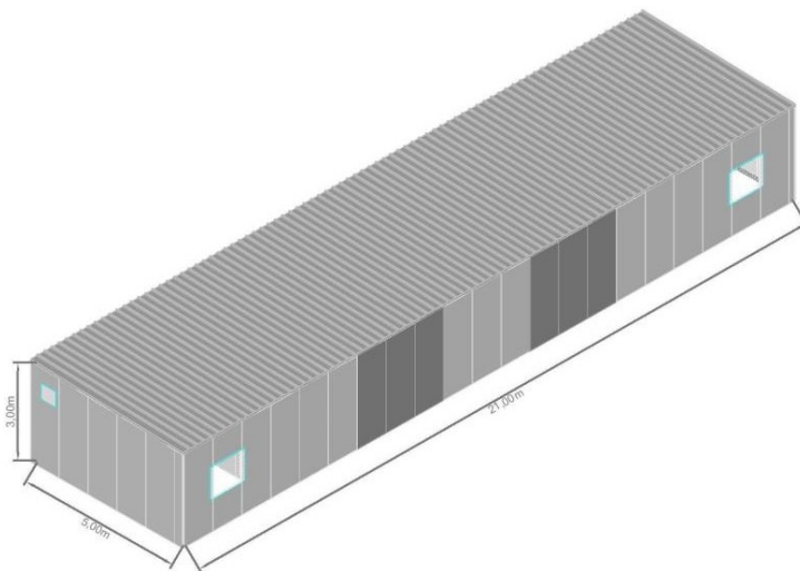
Σχέδιο 1. Διαστάσεις οικίσκου.
