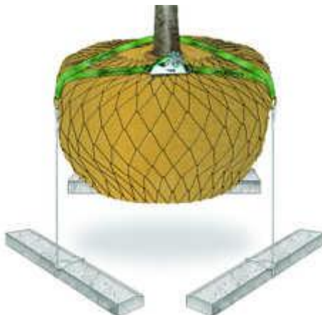
Εικόνα 2. Σύστημα υποστήλωσης ενδεικτικού τύπου “Platirus Deadman – Ιμάντας”
