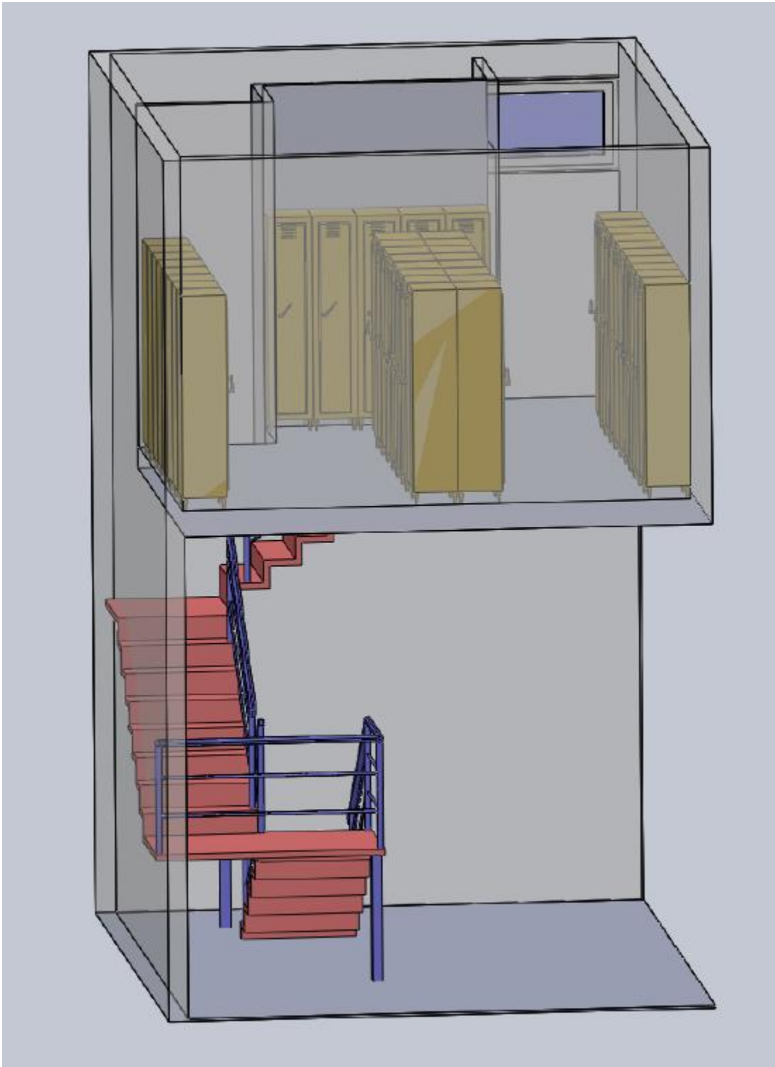
Αποδυτήρια. Σχέδιο 6
