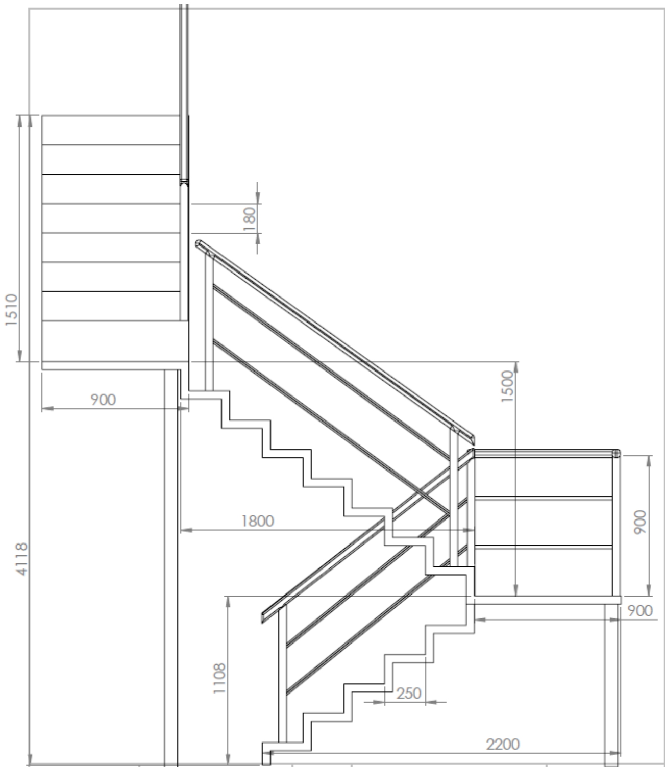
Κλίμακα. Σχέδιο 3
